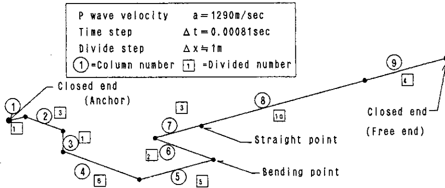
図 24 流路の分割と計算パラメータ Fig. 24 Divided fluid column number and calculation parameter for fluid response
