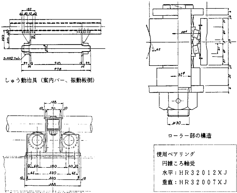
しゅう動治具（ローラーユニット、反力架構側）
