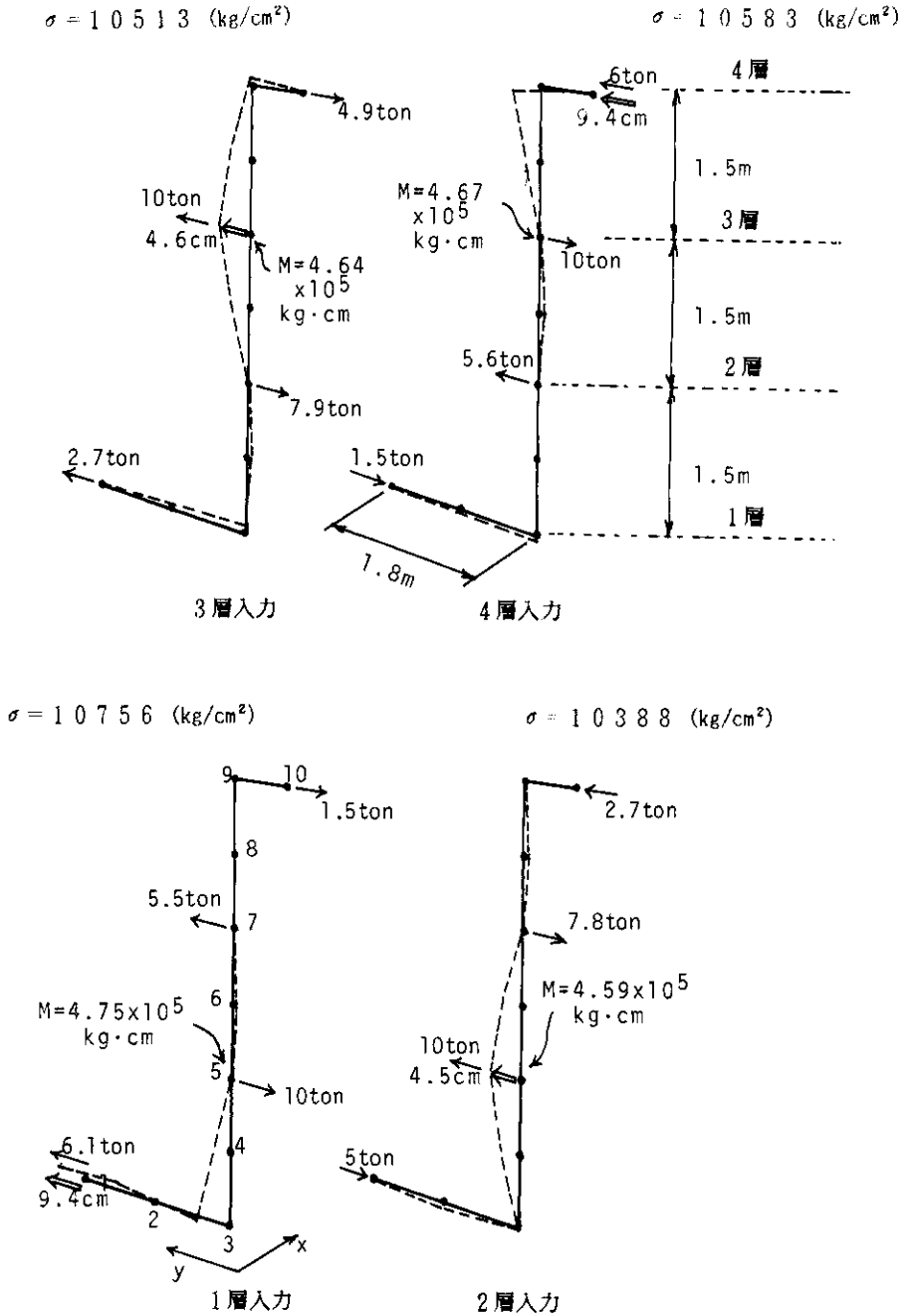
図 1.24 加振機の限界能力 (10 ton、±15 cm) における配管の静変形と応力 (4B-Sch 20) Fig. 1.24 Pipe deformation and stress at limit performance of the actuators
