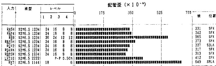
図 A.10 条件別多入力応答の比較（最大応答歪）
