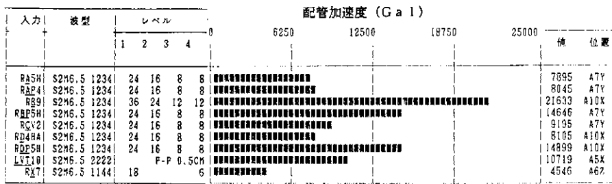
図 A.9 条件別多入力応答の比較（最大加速度）
