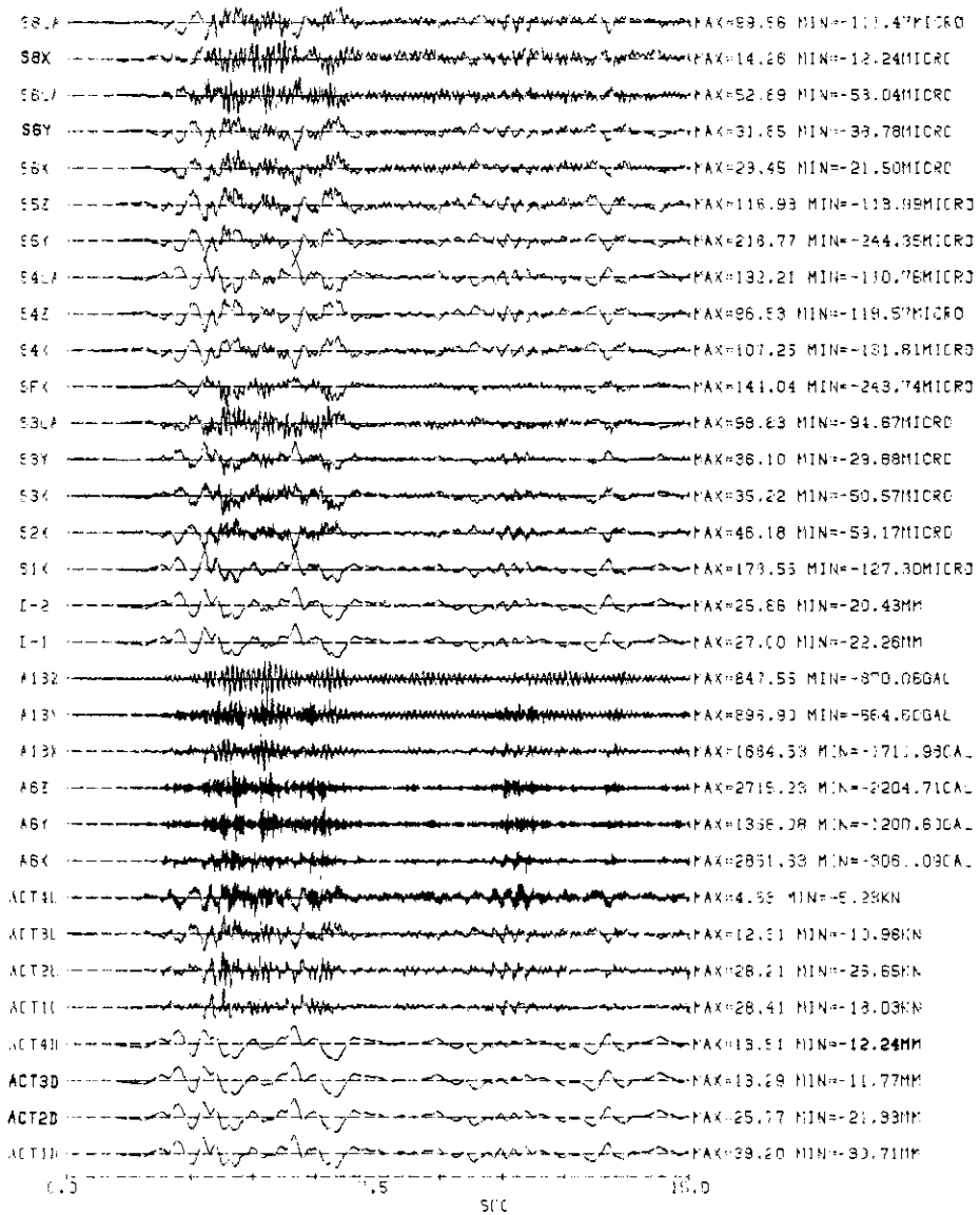
(a) E L N S 波 (動的多入力応答)
