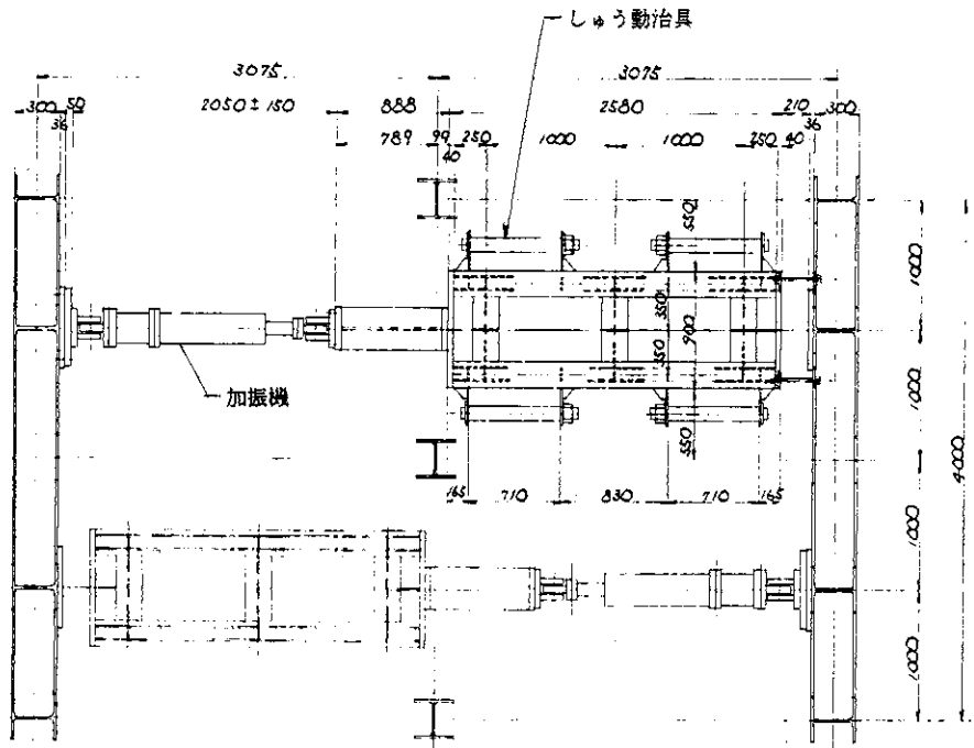
図 1.10 振動板構造概要
