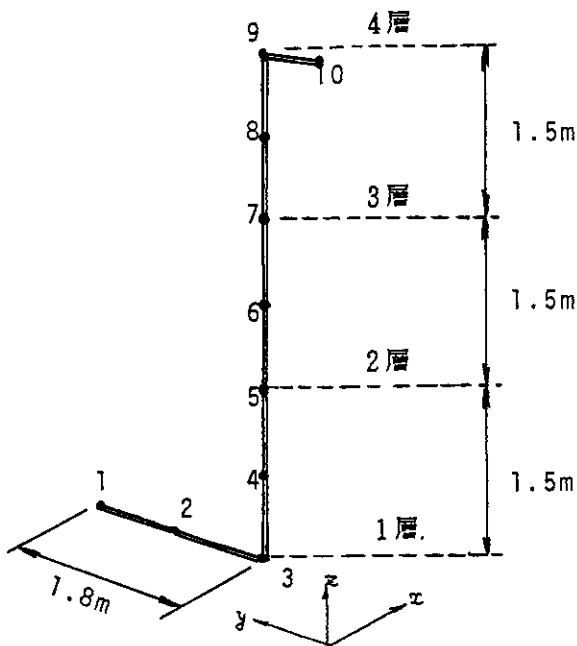
図 1.22 静的試験能力算定モデル
