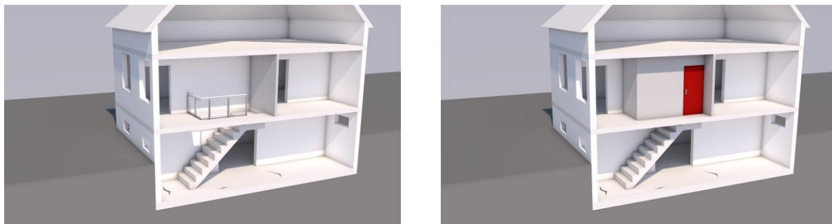
Abbildung 11: Gebäude mit einem offenen Treppenhaus zum Kellergeschoss (links), Gebäude mit einem gasdicht abgetrennten Treppenhaus zum Kellergeschoss (rechts)
