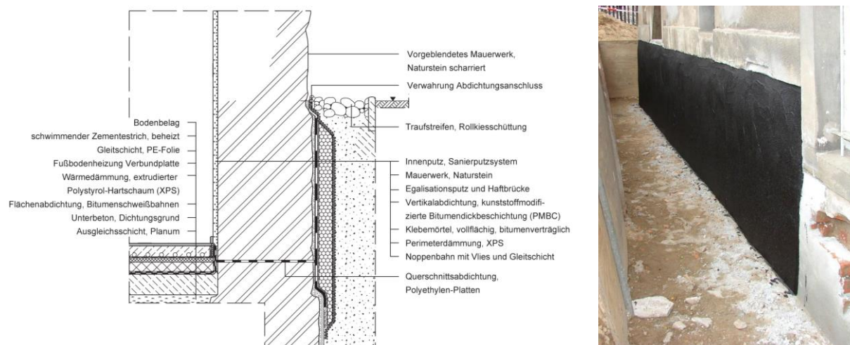
Abbildung 12: Beispielhafte Sanierungsplanung einer nachträglichen wannenartigen Abdichtungsstruktur an einem denkmalgeschützten Gebäude (links), nachträglich ausgeführte Vertikalabdichtung aus PMBC an einem denkmalgeschützten Gebäude (rechts), Quelle: GB1 Ingenieure
