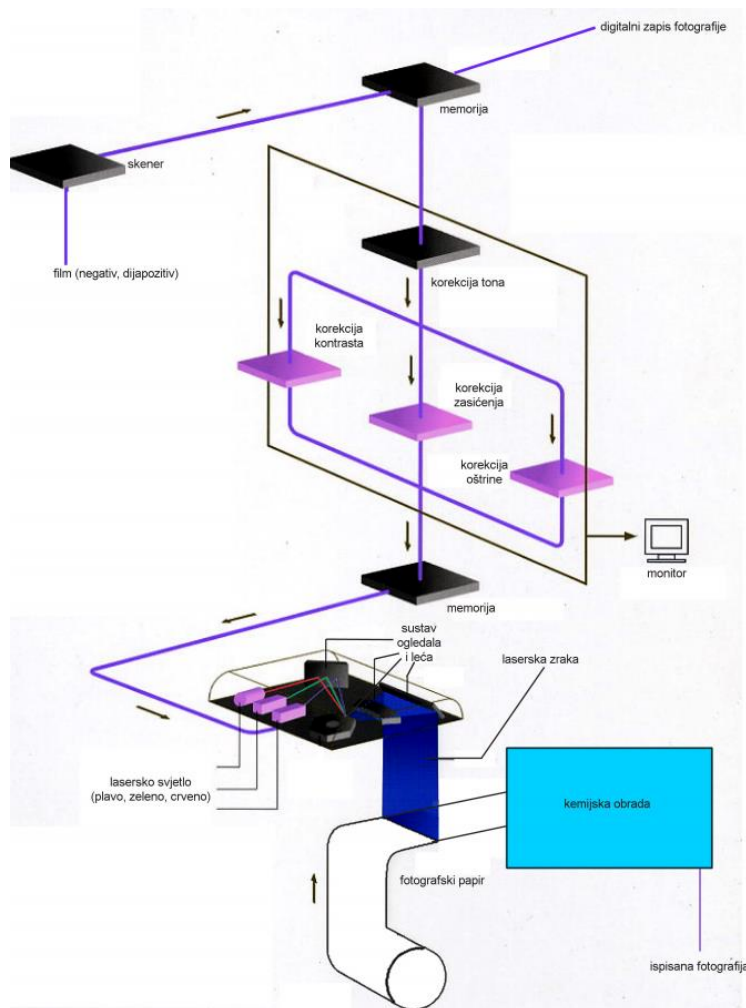
Slika 10. Princip rada laserskog digitalnih printera
