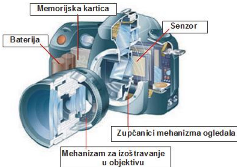
Slika 1. Digitalni fotoaparata
