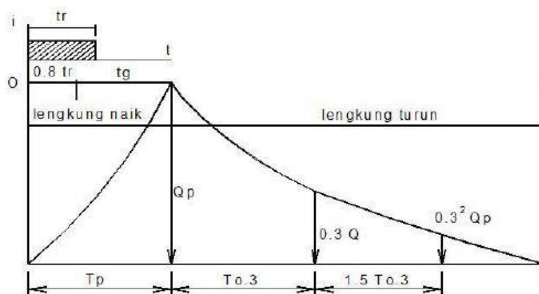
Gambar 3. Bentuk hidrograf dari satuan sintesis metode nakayasu
