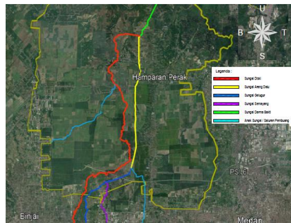
Gambar 7. Peta situasi sungai Diski
