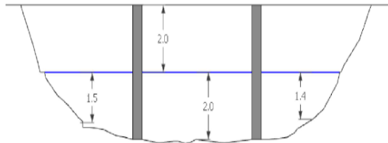
Gambar 6. Profil melintang sungai Diski
