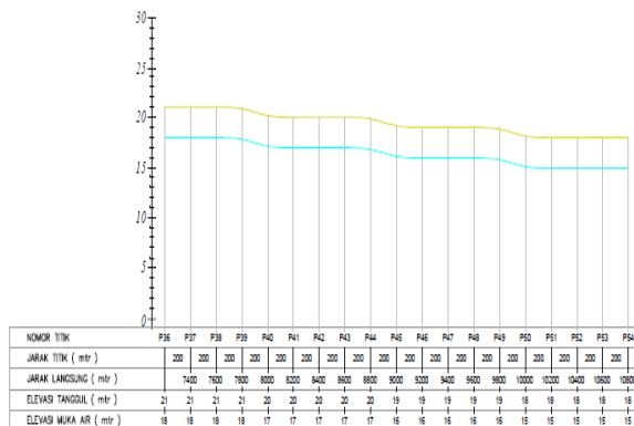
Gambar 5. Profil memanjang sungai diskki
