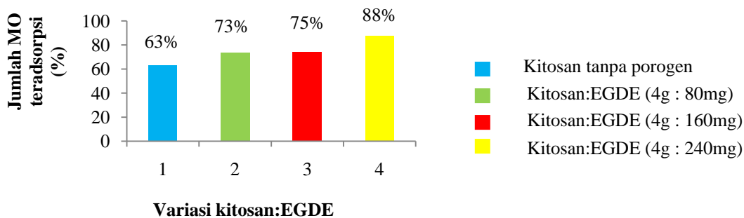
Gambar 3. Grafik hubungan variasi CS:EGDE terhadap jumlah methyl orange yang teradsorpsi pada CS-M
