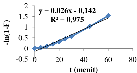
Gambar 5. Grafik hubungan waktu kontak ( t ) terhadap -\ln(1-F)
