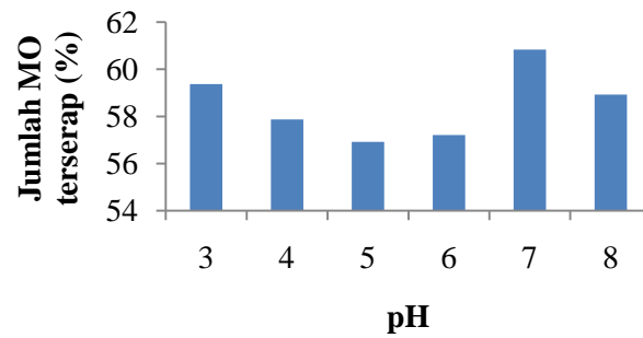
Gambar 2. Grafik hubungan pH terhadap jumlah methyl orange yang teradsorpsi pada CS-M
