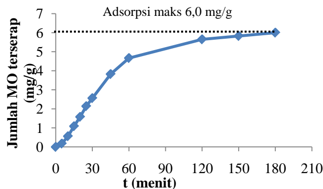
Gambar 4. Grafik hubungan waktu kontak terhadap jumlah methyl orange yang teradsorpsi pada kitosan makropori
