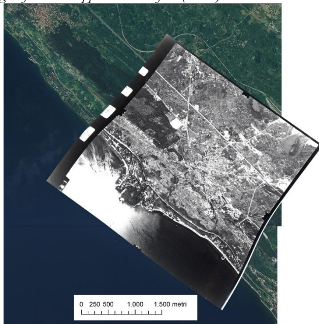
Fig. 3 – Distorsione dell'aerofotogramma IGM (1974) georiferito sovrapposto all'ortofoto (2007)
