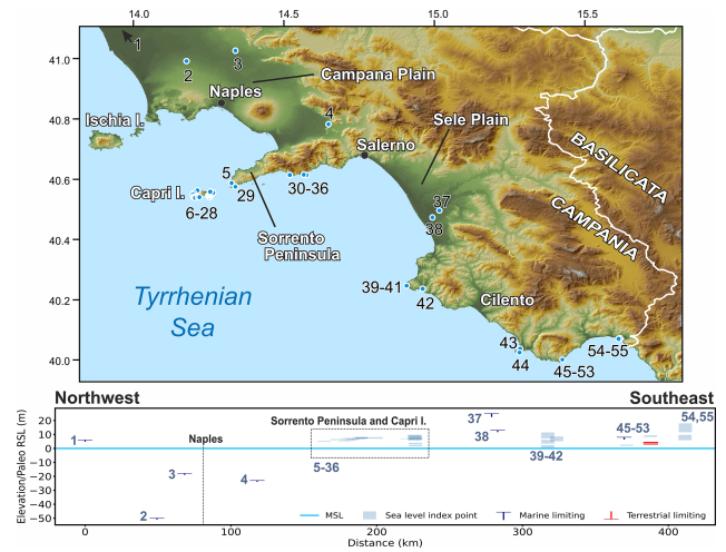
Figure 20. MIS 5 sea-level data for Campania (Italy). Upper panel: map of sites. The topography has been obtained from the SRTM void-filled DEM (Farr et al., 2007, NASA dataset). Lower panel: distance/elevation graph, from northwest (left) to southeast (right). Sites list: 1: Cellole Aurunci Masseria Transitiello (RSL ID 3624); 2: San Marcellino well (RSL ID 722); 3: San Marco Evangelista (RSL ID 739); 4: Sarno well (RSL ID 790); 5: Mitigliano (RSL ID 3581); 6: Scoglio Ricotta (I) Capri (RSL ID 821); 7: Scoglio Ricotta (II) Capri (RSL ID 822); 8: Grotta Testa del Cavallo Capri (RSL ID 800); 9: Grotta Jannarella Capri (RSL ID 801); 10: P.ta Campitiello Capri (RSL ID 802); 11: Cala del Limmo Capri (RSL ID 803); 12: Cala Articola (II) Capri (RSL ID 805); 13: Cala Articola (I) Capri (RSL ID 804); 14: Cala Articola (III) Capri (RSL ID 806); 15: Grotta Verde (I) Capri (RSL ID 807); 16: Grotta Verde (II) Capri (RSL ID 808); 17: Gr. Belvedere Capri (RSL ID 809); 18: Gr. Fontolina Capri (RSL ID 810); 19: I Faraglioni Capri (RSL ID 811); 20: Porto di Tragara (I) Capri (RSL ID 812); 21: Porto di Tragara (II) Capri (RSL ID 813); 22: P.ta di Masullo Capri (RSL ID 814); 23: a vascio funno Capri (RSL ID 815); 24: Cala Matermiana Capri (RSL ID 816); 25: Gr. Bianca (I) Capri (RSL ID 817); 26: Gr. Bianca (II) Capri (RSL ID 818); 27: P.ta della Chiavica Capri (RSL ID 819); 28: P.ta del Monaco Capri (RSL ID 820); 29: Cala di Ieranto (RSL ID 721); 30: Vettica Maggiore (RSL ID 823); 31: Grotta dello Smeraldo (RSL ID 798); 32: Conca dei Marini (III) Site I (RSL ID 767); 33: Conca dei Marini (II) Site I (RSL ID 766); 34: Conca dei Marini (I) Site I (RSL ID 720); 35: Conca dei Marini (V) (RSL ID 3623); 36: Conca dei Marini (IV) Site I (RSL ID 3565); 37: Ponte Barizzo (RSL ID 769); 38: Gromola (RSL ID 770); 39: Licosa Cape (III) (RSL ID 728); 40: Licosa Cape (II) (RSL ID 727); 41: Licosa Cape (I) (RSL ID 726); 42: Ogliastro Marina Baia Arena (RSL ID 592); 43: Palinuro Lido Ficocella (RSL ID 593); 44: Palinuro Cape (RSL ID 732); 45: The Riparo Infreschi cave (I) (RSL ID 3568); 46: The Riparo Infreschi cave (II) (RSL ID 3569); 47: The Riparo Infreschi cave (III) (RSL ID 3570); 48: The Riparo Infreschi cave (VI) (RSL ID 3573); 49: The Riparo Infreschi cave (IX) (RSL ID 3576); 50: The Riparo Infreschi cave (VIII) (RSL ID 3575); 51: The Riparo Infreschi cave (VII) (RSL ID 3574); 52: The Riparo Infreschi cave (V) (RSL ID 3572); 53: The Riparo Infreschi cave (IV) (RSL ID 3571); 54: Sapri (II) (RSL ID 792); 55: Sapri (RSL ID 791).
