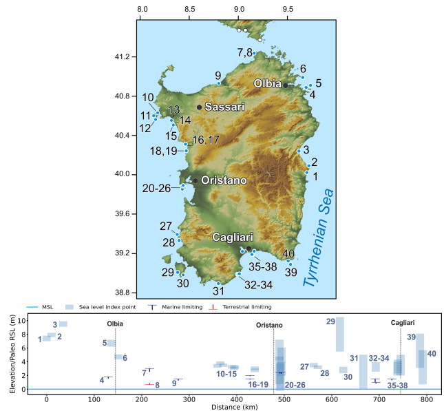
Figure 31. MIS 5 sea-level data for Sardinia (Italy). Upper panel: map of sites. The topography has been obtained from the SRTM void-filled DEM (Farr et al., 2007, NASA dataset). Lower panel: distance/elevation graph, counterclockwise around the island. Sites list: 1: Pedralonga (RSL ID 432); 2: Capo Monte Santu (RSL ID 435); 3: Orosei Nord (RSL ID 434); 4: Tavolara Punta la mandria (RSL ID 292); 5: Tavolara (RSL ID 431); 6: Capo Figari (RSL ID 430); 7: Capo Testa, Santa Reparata TLI (RSL ID 289); 8: Capo Testa, Santa Reparata MLI (RSL ID 290); 9: Badesi Mare San Pietro a Mare (RSL ID 300); 10: Cala Viola (RSL ID 388); 11: Capo Caccia 1 (RSL ID 382); 12: Capo Caccia 2 (RSL ID 383); 13: El tró (RSL ID 234); 14: Punta Padre Bellu (RSL ID 235); 15: Baurantinu (RSL ID 236); 16: Bosa Sect.1 (RSL ID 241); 17: Bosa Sect 2 (RSL ID 243); 18: Bosa Sect 3 (RSL ID 244); 19: Porto Alabe (RSL ID 238); 20: San Giovanni del Sinis (RSL ID 262); 21: San Giovanni del Sinis (RSL ID 271); 22: San Giovanni del Sinis (RSL ID 272); 23: San Giovanni del Sinis (RSL ID 265); 24: Faro Capo San Marco (RSL ID 266); 25: Capo San Marco (RSL ID 261); 26: San Giovanni del Sinis (RSL ID 263); 27: Buggerru (RSL ID 437); 28: Masua (RSL ID 436); 29: Sant'Antioco Cala Sapone (RSL ID 296); 30: Sant'Antioco (RSL ID 433); 31: Capo Malfatano (RSL ID 295); 32: Nora (RSL ID 1336); 33: Nora Is Fradis (RSL ID 1337); 34: Nora-Is Fradis (RSL ID 279); 35: Sa Illetta (RSL ID 278); 36: Cagliari Marina Piccola (RSL ID 1338); 37: Cagliari Cala Mosca (RSL ID 132); 38: Is Arenas (RSL ID 276); 39: Capo Carbonara Villasimius (RSL ID 293); 40: Capo Carbonara Isola dei cavoli-Cala Ponente (RSL ID 294).
