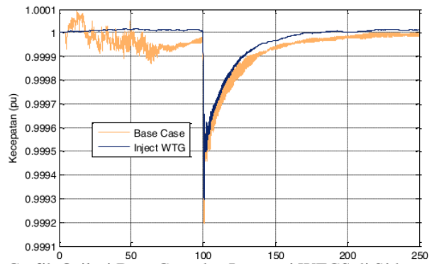
Gambar 4.13 Grafik Osilasi Base Case dan Integrasi WECS di Sidrap dan Jenepono pada Shaft Generator Low Pressure
