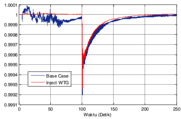
Gambar 4. 10 Grafik Kecepatan Base Case dan Integrasi WECS di Jeneponto pada Shaft Generator Low Pressure
