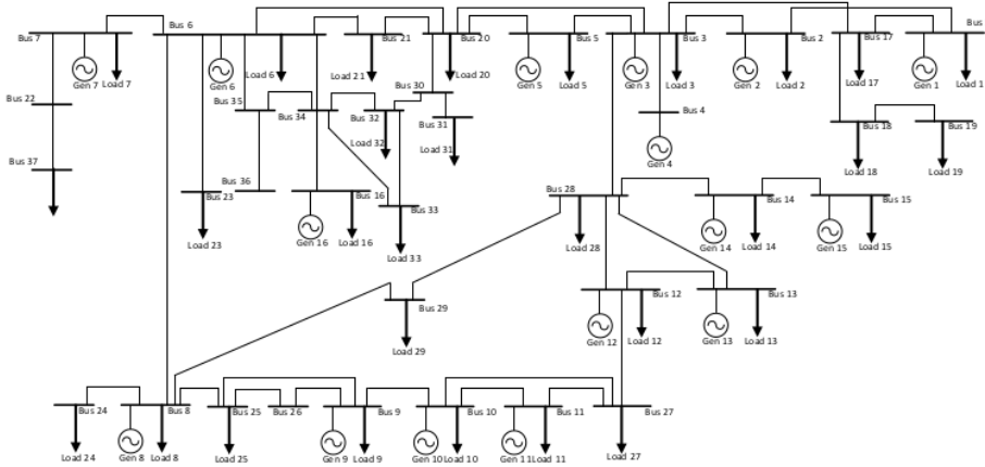
Gambar 3.1 Sistem Kelistrikan Sulselbar.
