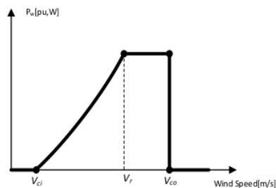
Gambar 2.2. Kurva Karakteristik Turbine Angin.
