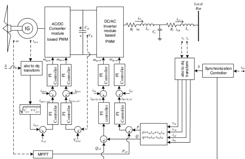
Gambar 2.3. Model Dinamik dari PLTB berbasis FRC.
