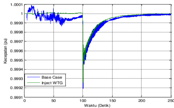
Gambar 4. 7 Grafik Kecepatan Base Case dan integrasi WECS di Sidrap pada Shaft Generator Intermediate Pressure
