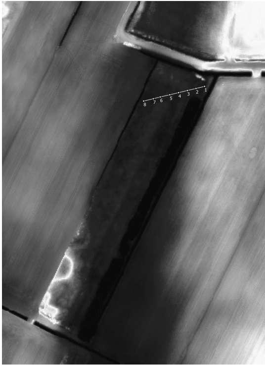
Abb. 3 Digitales Geländemodell der Restrinne der „verschwundenen Ems“ beim „Harener Wäldchen“. Unten links die Reste einer flussbegleitenden Düne, erkennbar an den hellen Farbtönen.
