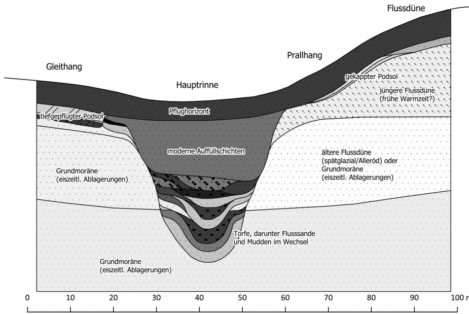
Abb. 4 Aus den Bohrdaten konstruiertes, 20fach überhöhtes Profil durch die „verschwundene Ems“ bei Landegge, Blick quer zum Ver- lauf bzw. von SO.
