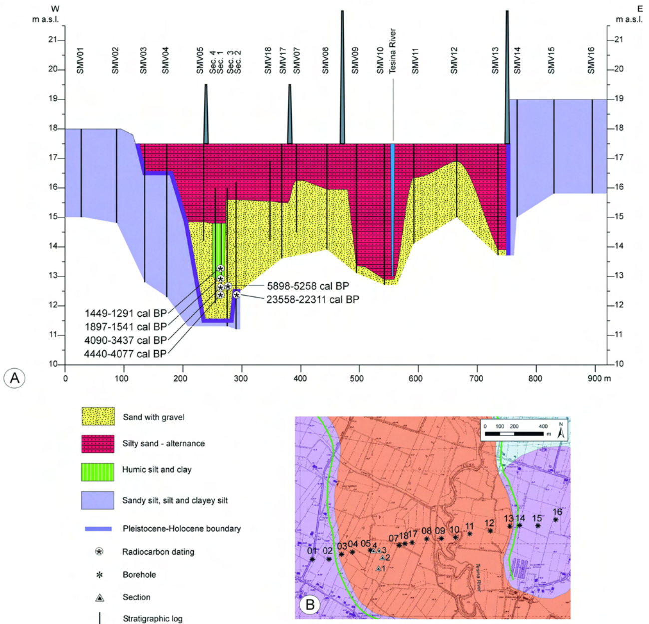
Fig. 7 – SM Veggiano cross section (A) and location map (B). Profilo stratigrafico di SM Veggiano (A) e sua ubicazione (B).
