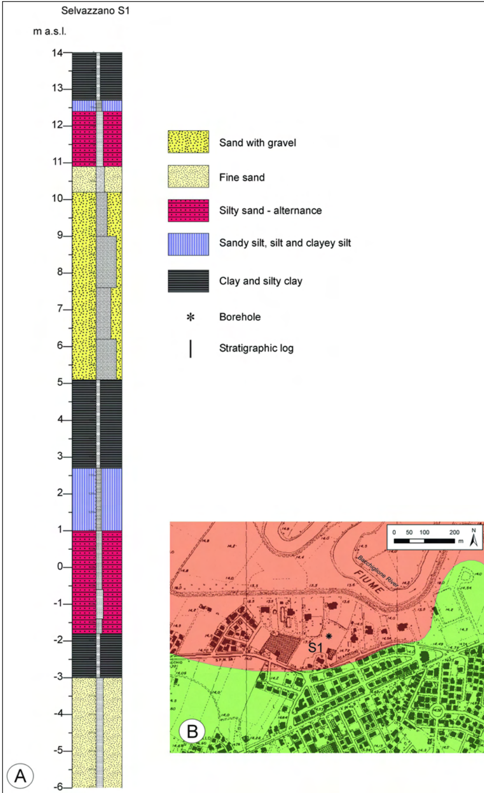
Fig. 8 - Stratigraphic log of S1 borehole at Selvazzano Dentro (A) and location map (B). Log stratigrafico del sondaggio S1 a Selvazzano Dentro (A) e sua ubicazione (B).
