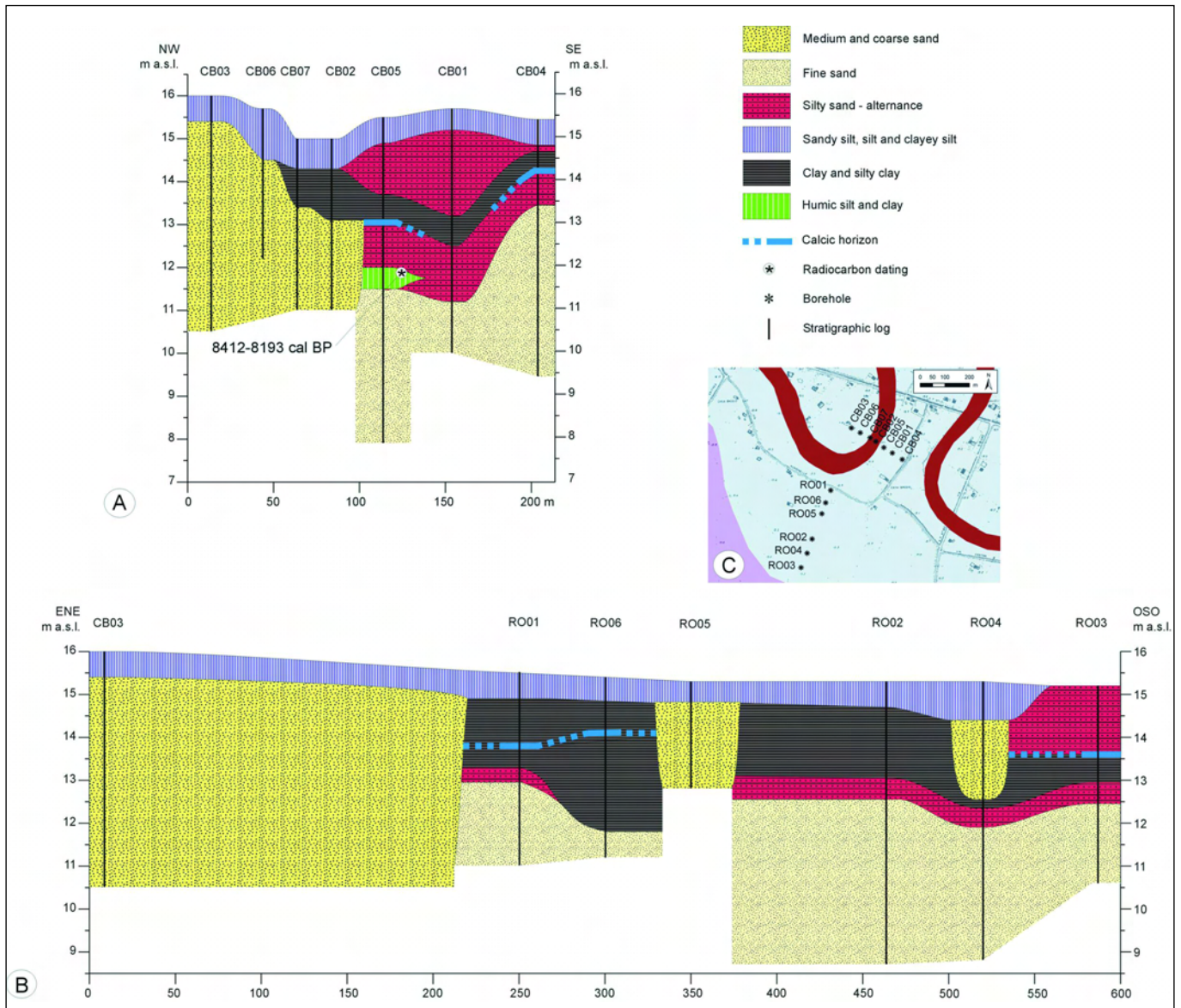
Fig. 3 - Ca' Baggio (A) and Rondinelle (B) cross sections and location map (C). Sezioni stratigrafiche di Ca' Baggio (A) e Rondinelle (B) e loro ubicazione (C).
