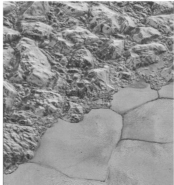
9. ábra: A New Horizons-szonda képe a Plútóról. A jobb oldali fotó a „tengerpartot” mutatja. Itt a síkvidék (jobb alsó sarok) a metán-tenger jege, amelynek összeáramlási vonalait jelzik a lineamentumok. A parton kívüli sziklák anyaga vízjég lehet.
