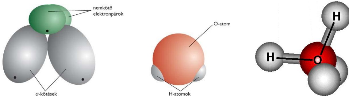
1. ábra: A vízmolekula négy elektronpárja, az oxigén és a hidrogén atomok elhelyezkedése ( 104^\circ -os szög).
