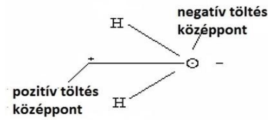
2. ábra: A dipólus szerkezetű vízmolekula.
