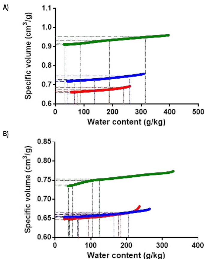
Figure 2. Specific volume as a function of soil water content for quasi-pristine (QP), integrated crop/livestock (ICL) and continuous cropping (CC) treatments for two soil types: Argiudoll (A) and Hapludoll (B). Figura 2. Volumen específico en función del contenido hídrico del suelo para los tratamientos cuasi-prístino (QP), agrícola ganadera (ICL) y agricultura continua (CC), para dos tipos de suelos: Argiudol (A) y Hapludol (B).
