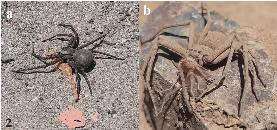
Figura 2. a. Hembra adulta de Sicarius thomisoides predando sobre un ejemplar de Brachistosternus mattoni en Mejillones, Región de Antofagasta. b. Hembra subadulta de S. thomisoides predando sobre un ejemplar de Pseudocleobis sp. en Llay-Llay, Región de Valparaíso. / Adult female of Sicarius thomisoides predating on a Brachistosternus mattoni specimen in Mejillones, Antofagasta Region. b. Subadult female of S. thomisoides predating on a specimen of Pseudocleobis sp. in Llay-Llay, Valparaíso Region.
