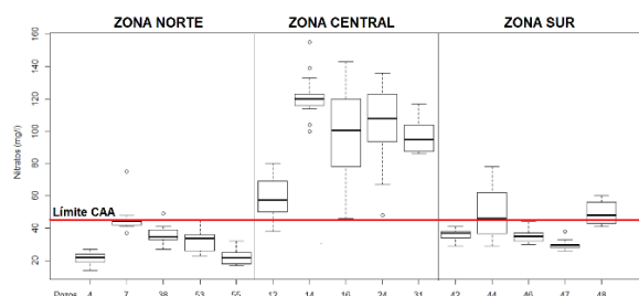
Figura 6. Diagramas bloxplot.
