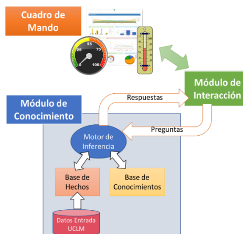
Figura 1. Arquitectura propuesta para la aplicación
