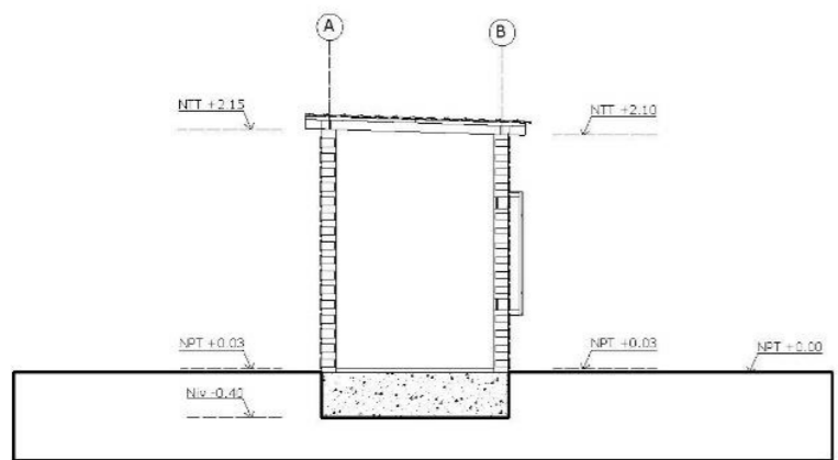
Corte A-A
