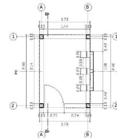
Planta General
