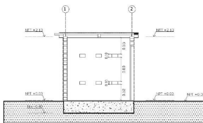
Corte B-B
