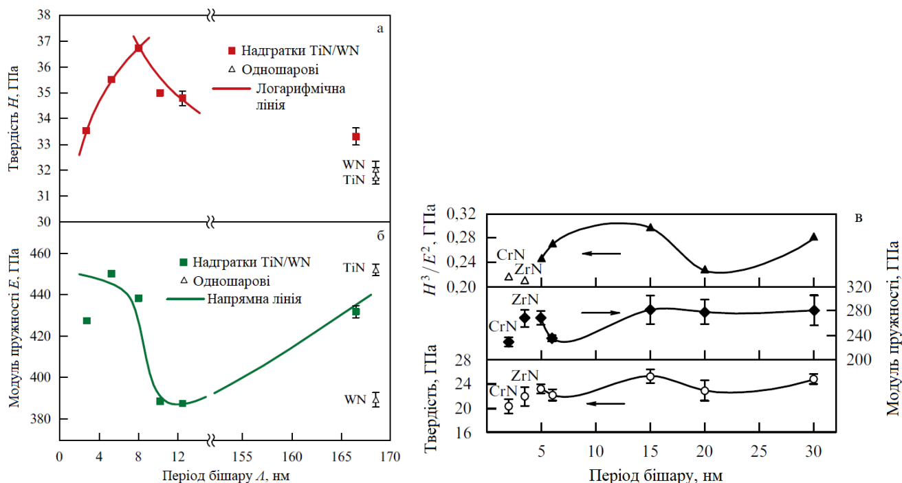
Рисунок 1.1 — Залежність твердості (а) і модуля пружності (б) від періоду бішару для надрешіток TiN/WN [58]. Твердість, модуль пружності та деформація в залежності від товщини бішару CrN/ZrN покриттів [57]
