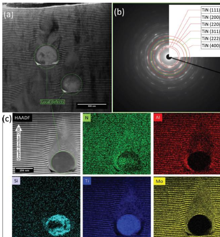
Рисунок 3.10—Зображення ПЕМ поперечного перерізу зони утворення дифузії (а), SAED зображення із зеленої пунктирної області (b) та відповідні ЕДС карти елементних розподілів (c) системи \text{TiAlSiYN}/\text{MoN} , осадженої на сталеву підкладку
