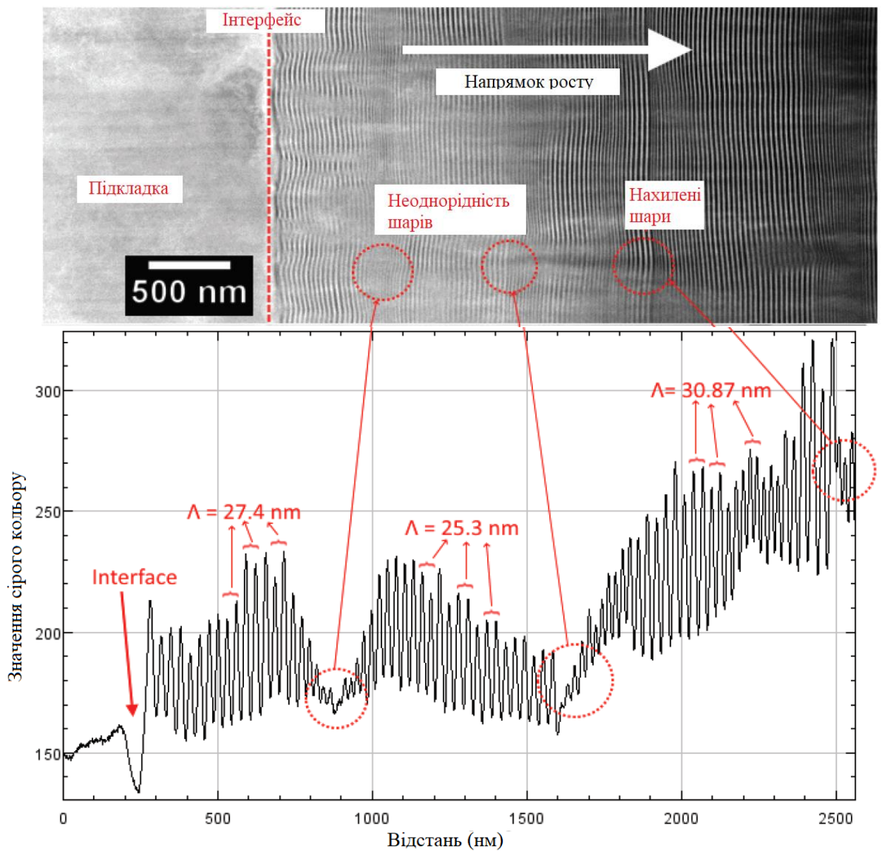
Рисунок 3.7 – ПЕМ-зображення поперечного перерізу багат шарової структури \text{TiAlSiYN}/\text{MoN} після осадження та відповідні лінійні сканування, що показують, як змінюється товщина шарів уздовж поперечного перерізу покриття
