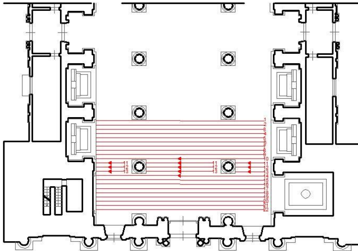
Figura 7 - Schema dei profili georadar.
