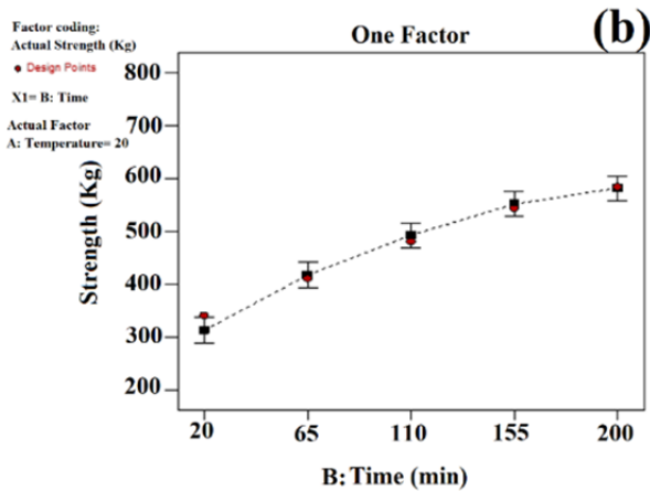
نمودار ۶ اثر مستقل پارامترهای دما و زمان پخت روی استحکام برشی: (a) دما، (b) زمان پخت
