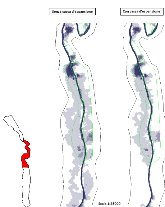
Figura 9b. Aree allagate nel tratto intermedio in assenza di cassa d'espansione e in sua presenza.
