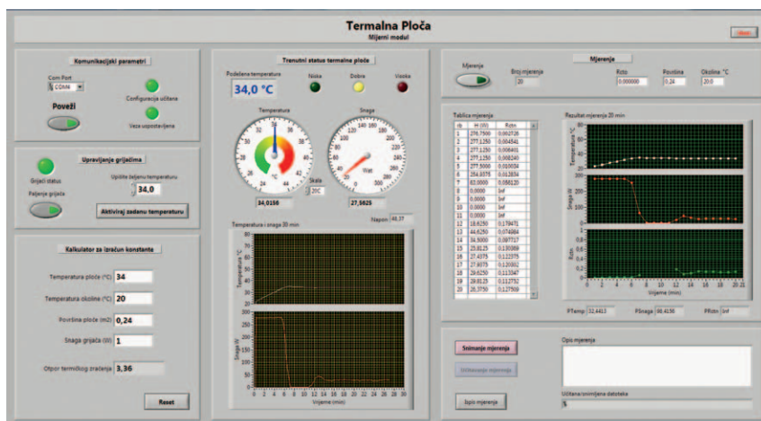
Sl.3 Zaslom računalnog programa za upravljanje i mjerenje parametara na vrućoj ploči
