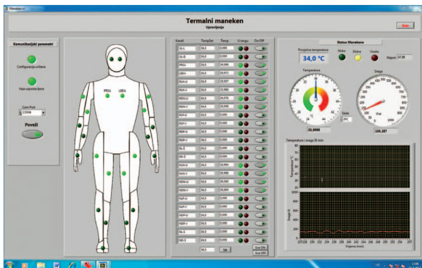
Sl.4 Zaslom računalnog programa za upravljanje parametrima na termalnom manekenu
