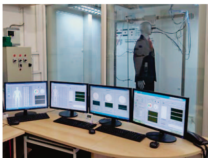
Sl.1 Mjerni sustav za određivanje statičkih i dinamičkih toplinskih svojstava kompozita i odjeće
