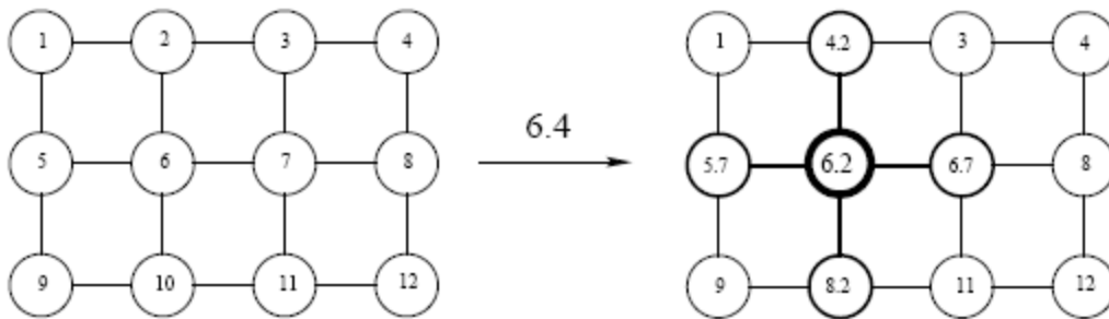
Figure 1: SOM training algorithm
