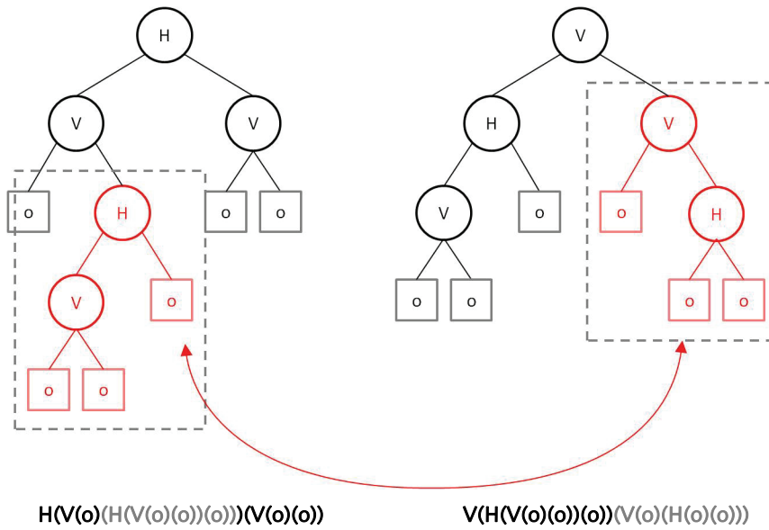
Abb. 14: Genetische Programmierung: Mutation eines Individuums durch Änderung der Unterteilungsrichtung
