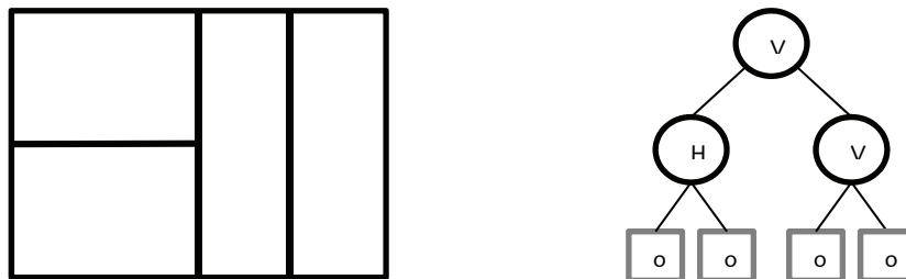
Abb. 4: Interpretation der Unterteilungssyntax V(H(o)(o))(V(o)(o)) bzw. des Slicing Floorplans (links) als Slicing Tree (rechts)
