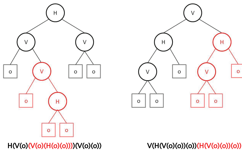
Abb. 15: Genetische Programmierung: Crossover von Ästen zwischen zwei Syntaxbäumen
