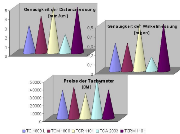
Abb.2 Vergleich tachymetrischer Systeme
