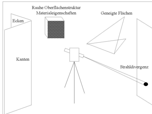
Abb. 3. Problemfelder bei der reflektorlosen Tachymetrie
