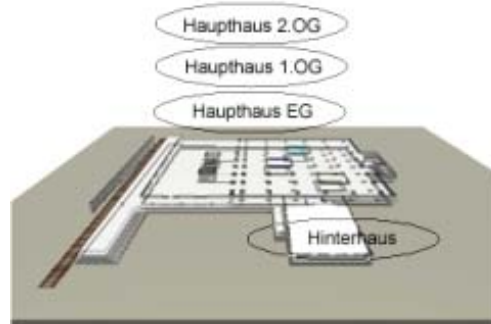
Abbildung 5 unterschiedliche Detaillierungsgrade
