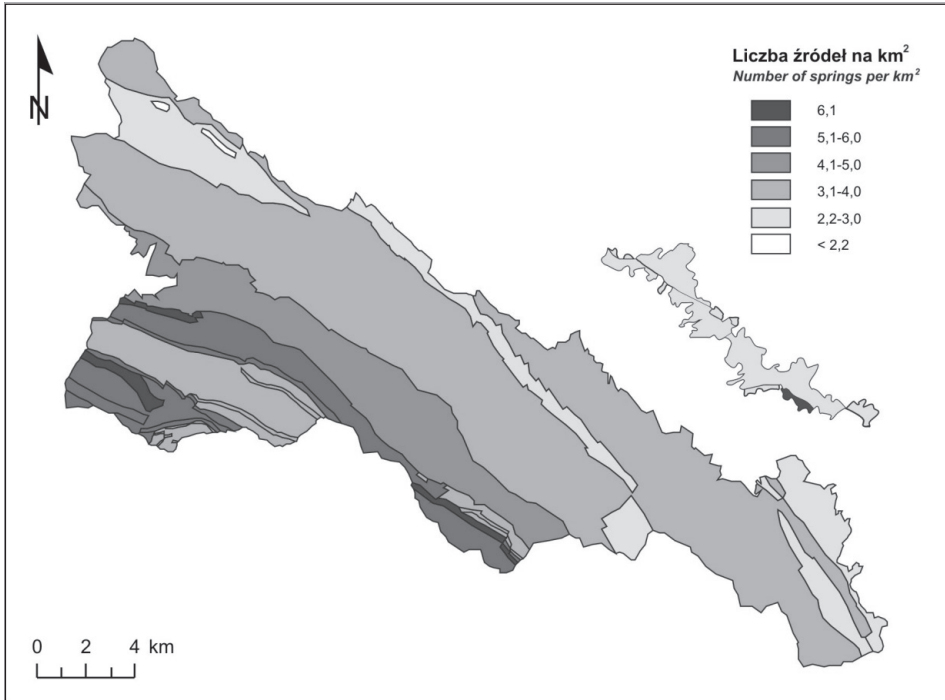
Ryc. 4. Wskaźnik krenologiczny poszczególnych jednostek strukturalnych na obszarze BdPN. Opracowanie własne na podstawie Łajczak 2010a, Łajczak 2010b i Tokarski 2010. Fig. 4. Spring density index within structural units in the Bieszczady National Park. Own elaboration based on Łajczak 2010a, Łajczak 2010b and Tokarski 2010.
