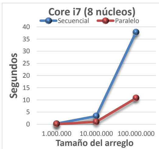
Figura 5. Comportamiento del MergeSort Computador Core i7
