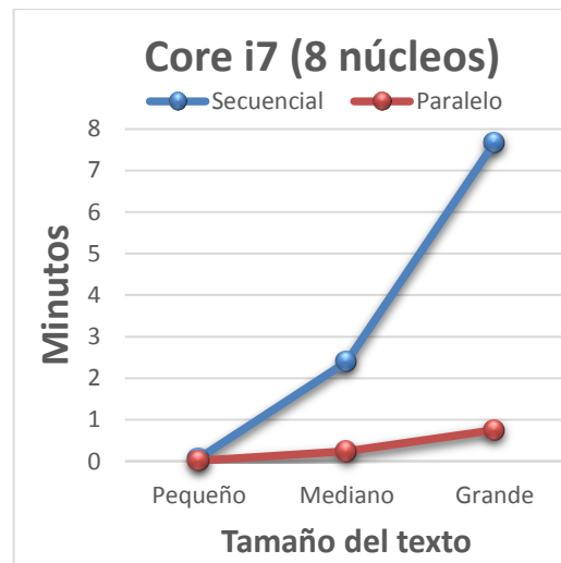
Figura 7. Comportamiento del método de encriptación de datos. Computador Core i7
