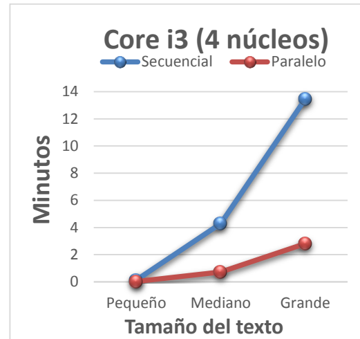
Figura 6. Comportamiento del método de encriptación de datos. Computador Core i3
