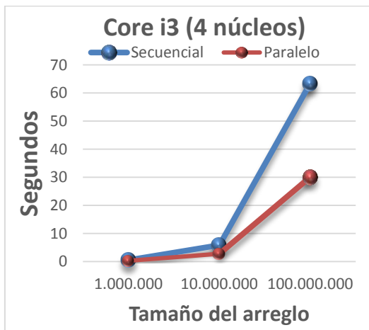
Figura 4. Comportamiento del MergeSort Computador Core i3
