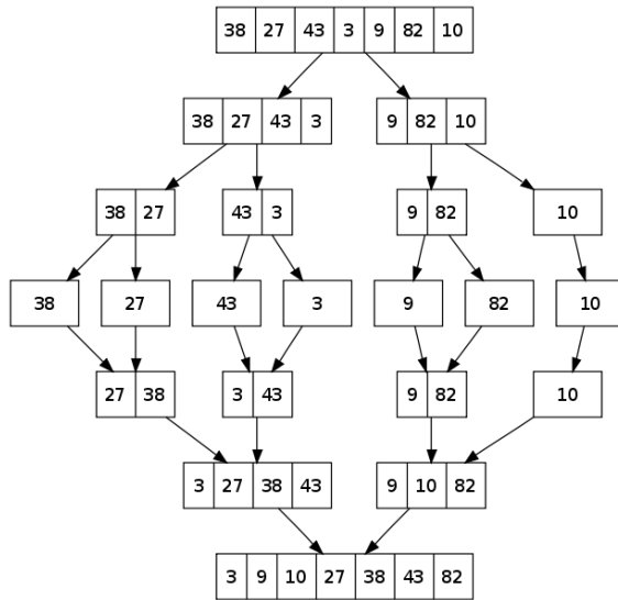
Figura 3. Ordenamiento MergeSort.
