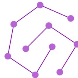
Рис. 7. Граф, состоящий из 10 вершин и 8 ребер
