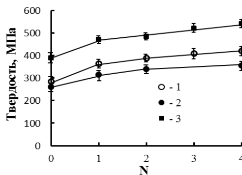
Рисунок - 5. Влияние числа РКУП на твердость спечённых КМ Al-Sn (2,3) и алюминиевой матрицы (1). Содержание олова, вес. %: 1,2 – 20, 3 – 40
