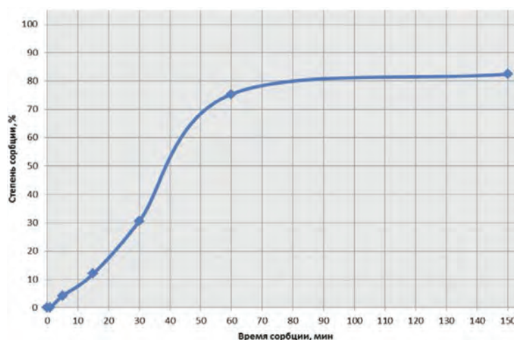
Рис. 1. Определение степени извлечения ионов As^{3+} из водного раствора с помощью исследуемого образца каталитического сорбента
