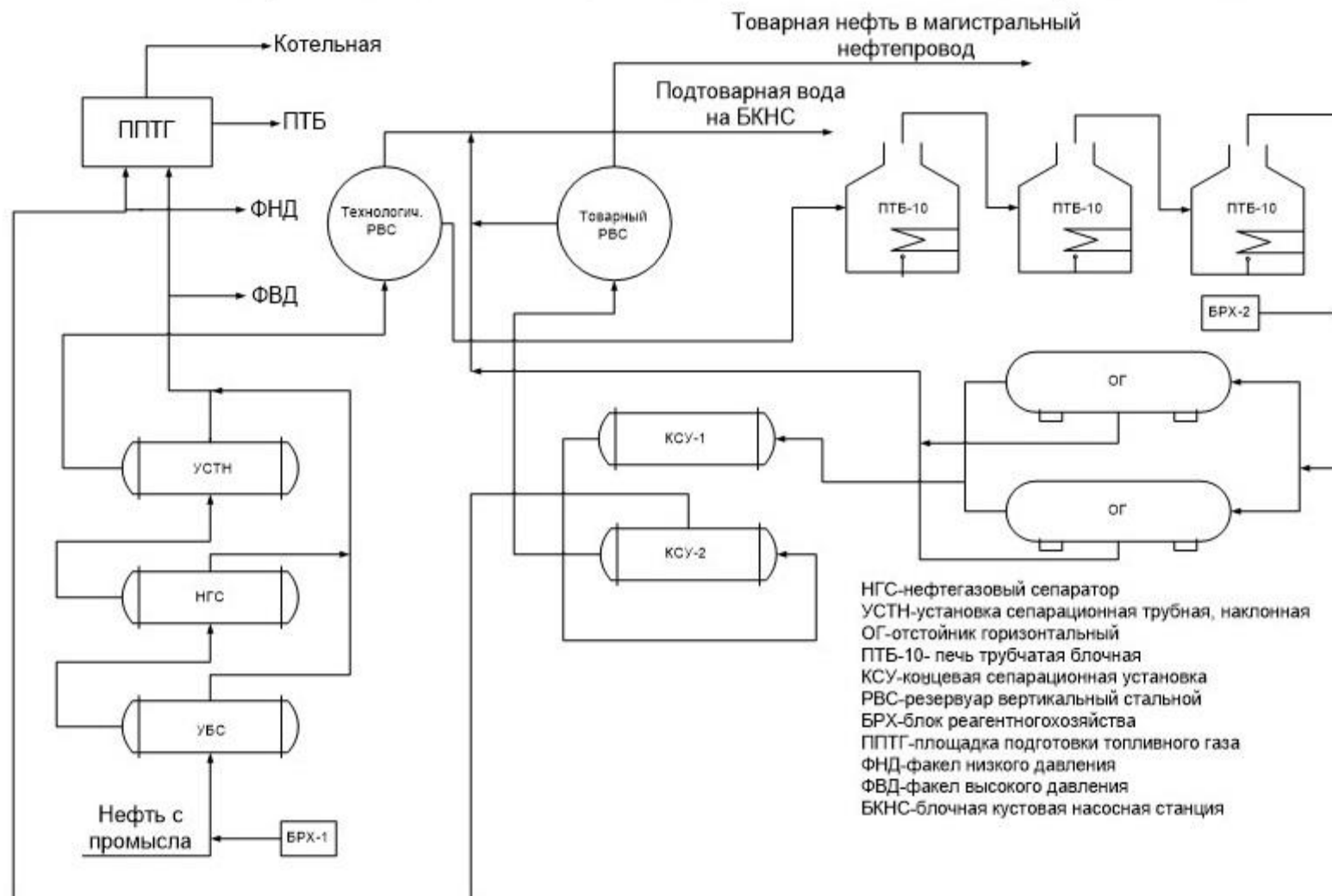
Рисунок 1.4 – Принципиальная технологическая схема ЦППН – 5 «Игол».
