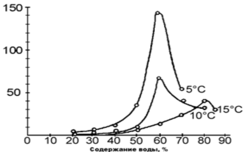
Рисунок 1.1 - Зависимость кажущейся вязкости эмульсии от содержания воды в нефти и температуры
