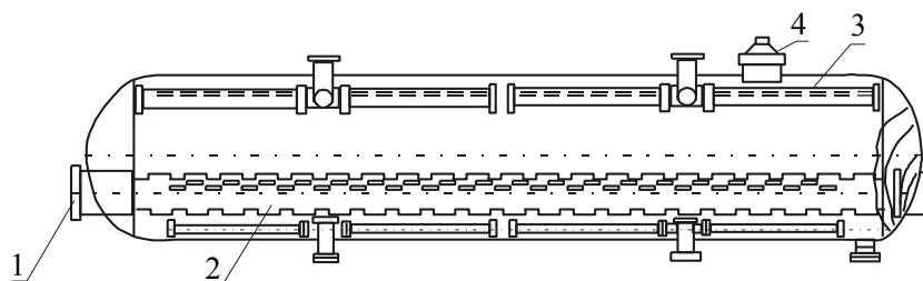
Рисунок 1.5 - Технологическая схема аппарата ОГ-200П для предварительного разделения нефти и пластовой воды
