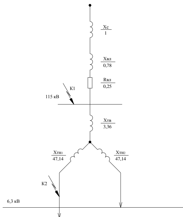
Рисунок 1. - Расчетная схема коротких замыканий в сетях выше 1 кВ. По расчетной схеме составляем схему замещения (рисунок 2)
