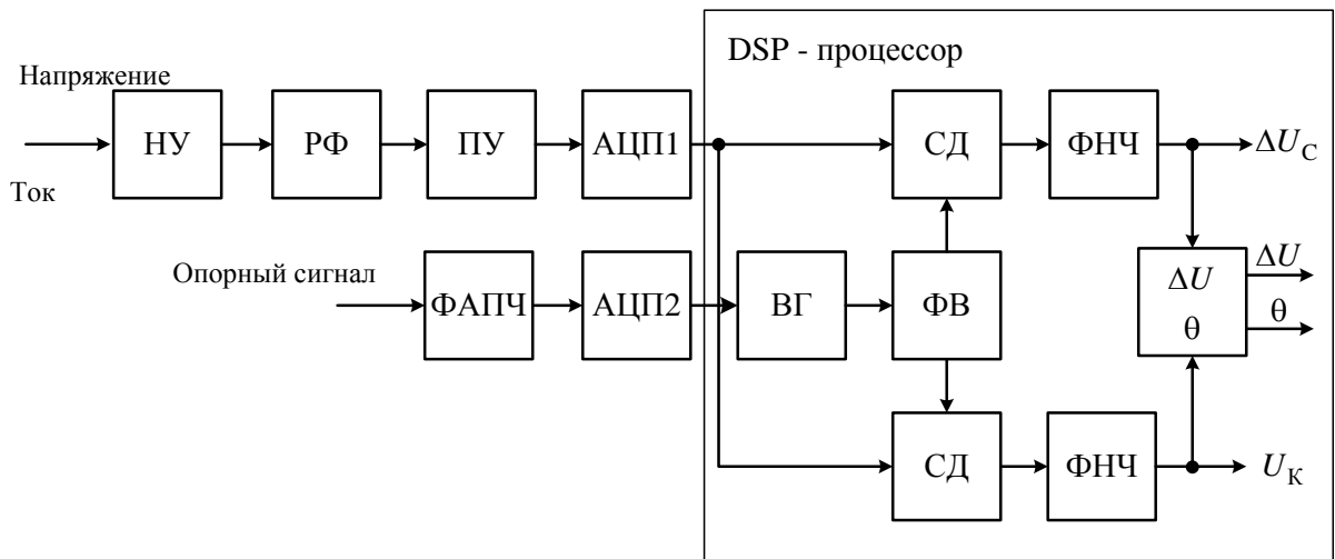
Рисунок 4 – Функциональная блок-схема типового синхронного усилителя
