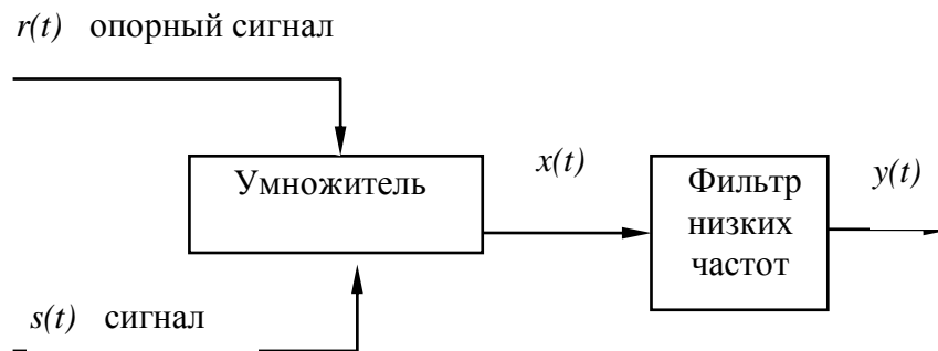
Рисунок 1 – Схема синхронного детектора
