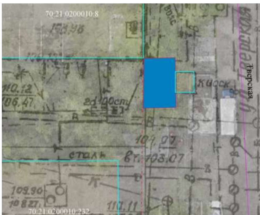
Рисунок 3 - Расположение инженерных коммуникаций
