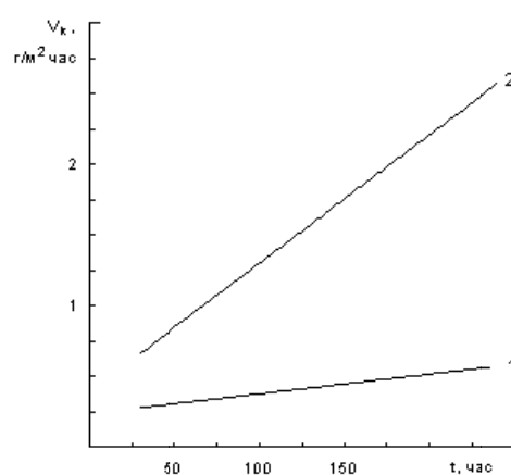
Рис. 6. Зависимость скорости коррозии от времени испытания после наплавки покрытий: 1) на постоянном токе, 2) импульсно - дуговым методом
