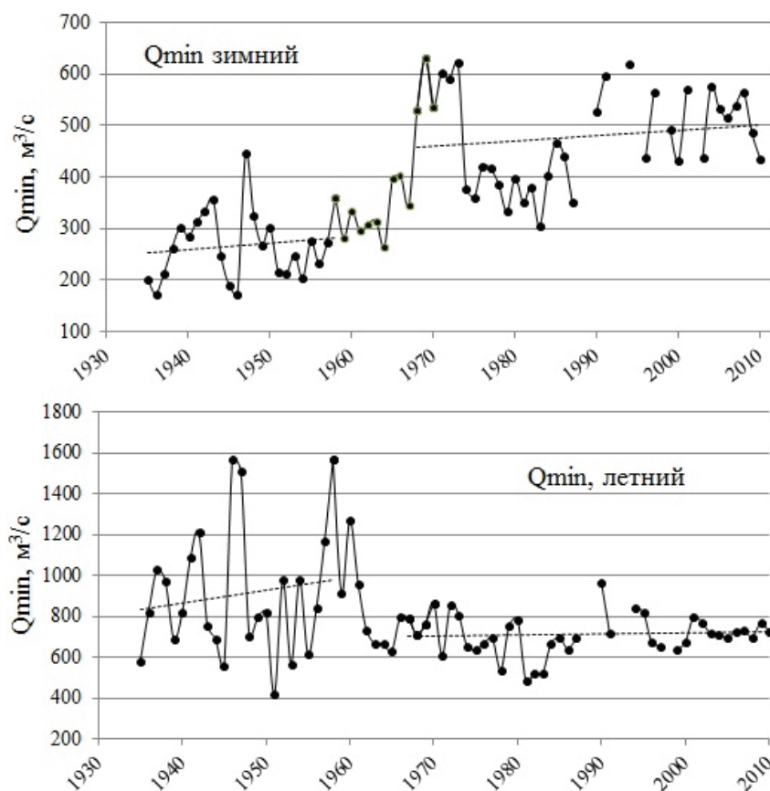
Рис. 2. Межгодовая динамика минимального среднемесячного стока р. Иртыш – п. Семиарка. Тенденции минимального стока, обозначенные пунктирной линией, статистически незначимы
