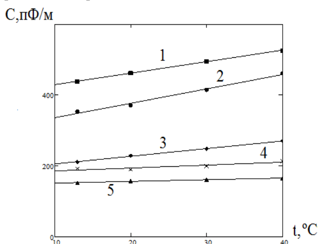
Рис. 3. «Зависимость влияния температуры воды на результат измерения погонной емкости»: 1- емкость кабеля С11, 2-емкость кабеля С14, 3-емкость кабеля С7, 4-емкость кабеля С10, 5-емкость кабеля С16
