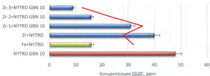
Рис. 1. Сравнительная диаграмма концентрации ДБДС при добавлении в трансформаторное масло железа (проба без нагревания) и циркония ( Zr+NYTRO GBN 10 – без нагревания, Zr-1+NYTRO GBN 10 – 100 °C в течение 1 часа, Zr-2+NYTRO GBN 10 – 100 °C, 12 часов, Zr-3+NYTRO GBN 10 – 100 °C, 48 часов )
