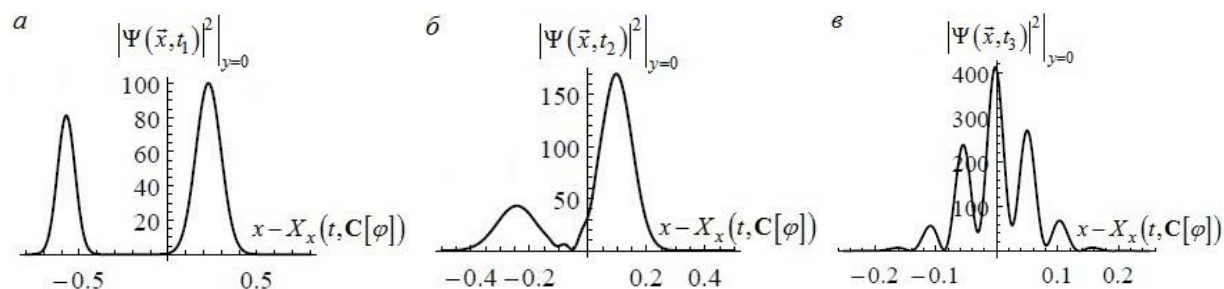
Рис. 1. |\Psi(x, t)|^2|_{y=0} для моментов времени t_1 = 0 (а); t_2 = 0,8 (б); t_3 = 1,1 (в)
