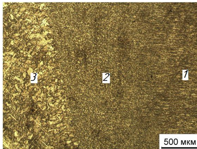
Рисунок 2 – приграничная область расплавленного металла (1 – основной металл с наноразмерными зёрнами; 2 – зона термического влияния; 3 – граничная область расплавленного металла)
