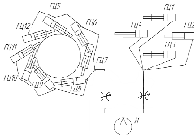
Рис. 2. Система регулирования подачи рабочей жидкости в гидроцилиндры стартового устройства ГЦ1-4 и гидроцилиндры поворота гехода ГЦ5-12 при помощи регулируемых дросселей
