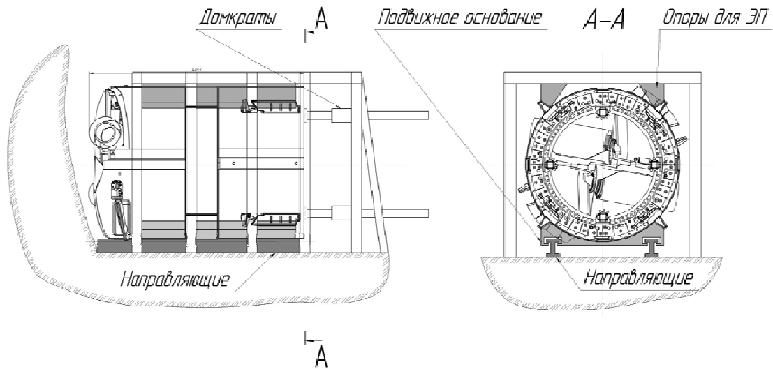
Рис. 1 Схема стартового устройства гехода
