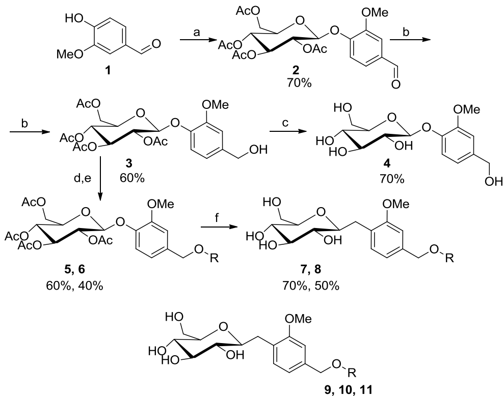
Рис. 2. Синтез целевых гликозидов: а) АБГ, Ag 2 O, ванилин, хинолин, 2ч; б) NaBH 4 , ЦТМАБ, CHCl 3 , H 2 O, 25-40°С, 4-6ч; в) MeOH, MeONa; д) PhOCl, 2 eq. Py, CHCl 3 , 24ч; е) RCl, 2 eq. Py, CHCl 3 , 24ч; ф) HCl/EtOH/CHCl 3 (3:1:1), 24ч.
