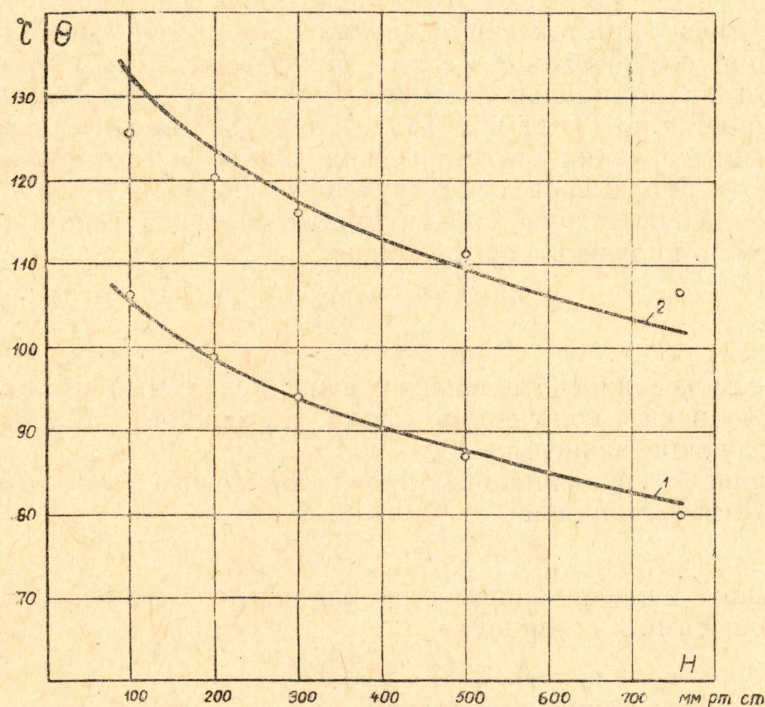
Рис 2. Зависимость средних перегревов корпуса и статорной обмотки синхронно-гистерезисного двигателя от атмосферного давления при \Sigma P_{const} . 1 — перегрев корпуса по (1) — (4), (6); 2 — перегрев статорной обмотки по (5); O — опытные значения перегревов.
