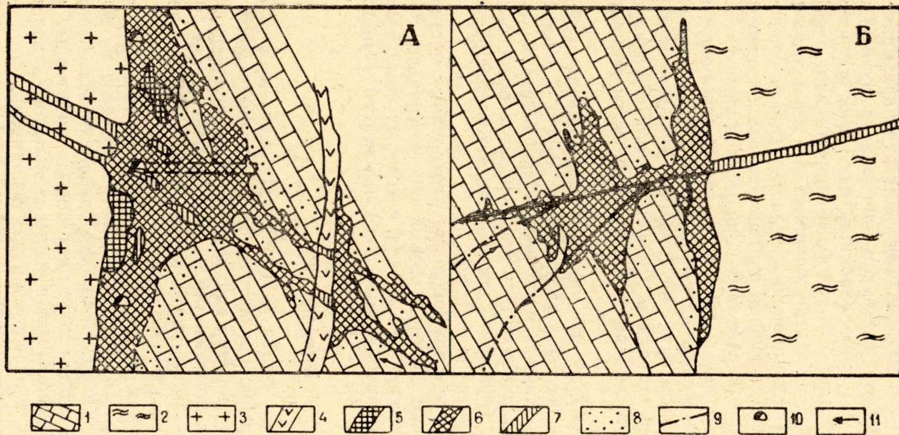
Рис. 3. Схема формирования контактовых рудных тел на пересечении рудной трещиной контактов карбонатных пород; А — с гранитами и дайками; В — с роговиками, на Ольховском месторождении (разрез). 1 — известняки и доломиты; 2 — роговики, ороговикованные эффузивно-сланцевые породы; 3 — граниты, гранодиориты; 4 — догранитные дайки диорит-порфиров; 5 — реликты карбонатно-пирротиновых руд 1-й стадии минерализации; 6 — массивные сульфидные руды (пирротин, пирит, халькопирит, марказит и др.); 7 — кварцевые, кварцево-сульфидные жилы; 8 — вкрапленные сульфидные руды; 9 — тектонические трещины; 10 — горные выработки; 11 — предполагаемое направление рудных растворов
