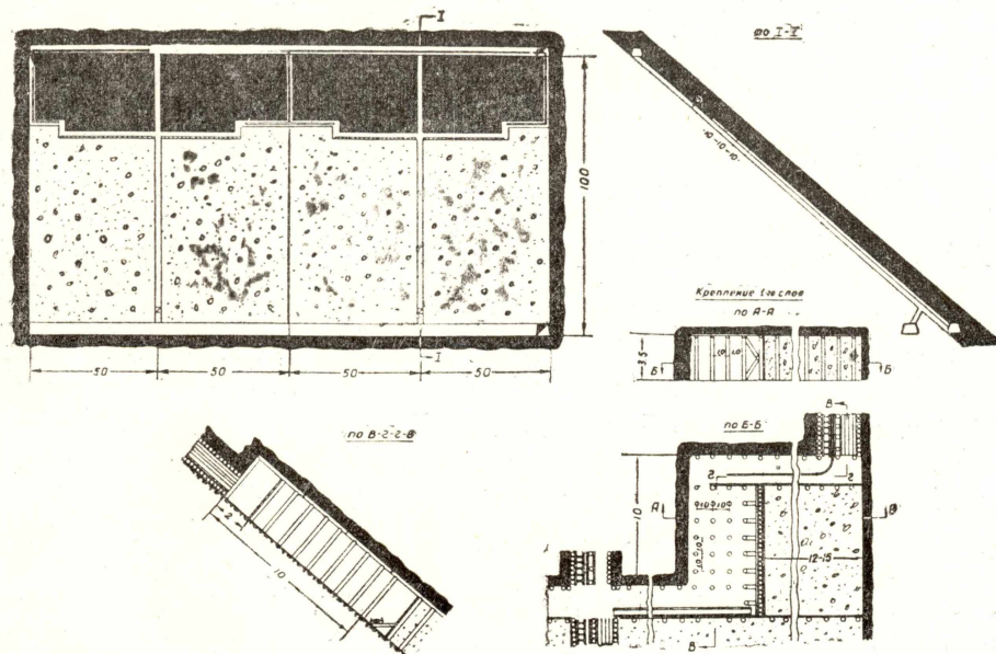
Рис. 10. Система разработки наклонными слоями с выемкой слоев полосами по простиранию
