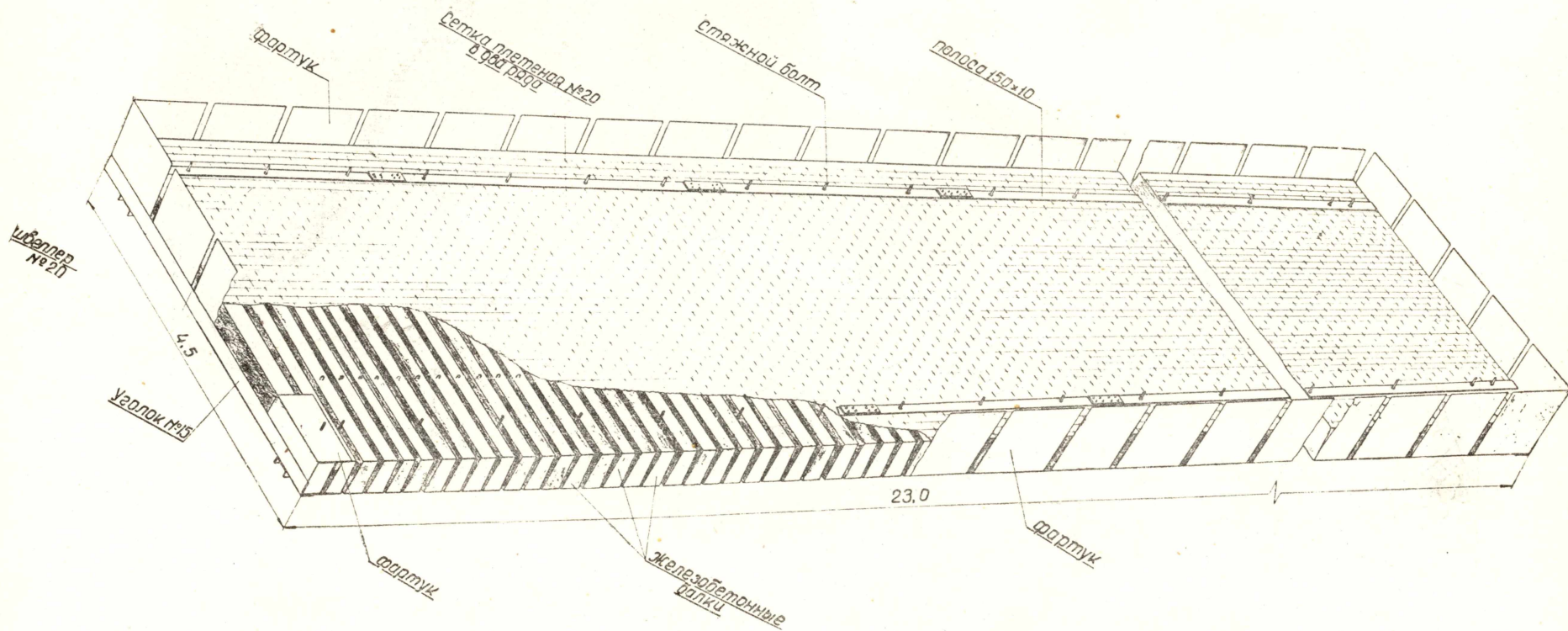
Рис. 3. Бессекционный эластичный щит из железобетонных балок
