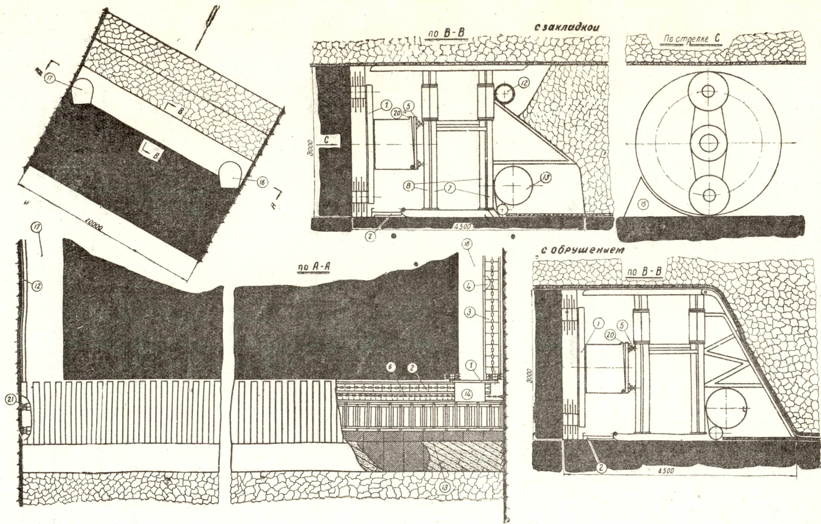
Рис. 9. Конструкция выемочно-крепильного агрегата «Кузбасс» для работы в условиях системы разработки поперечно-наклонными слоями
