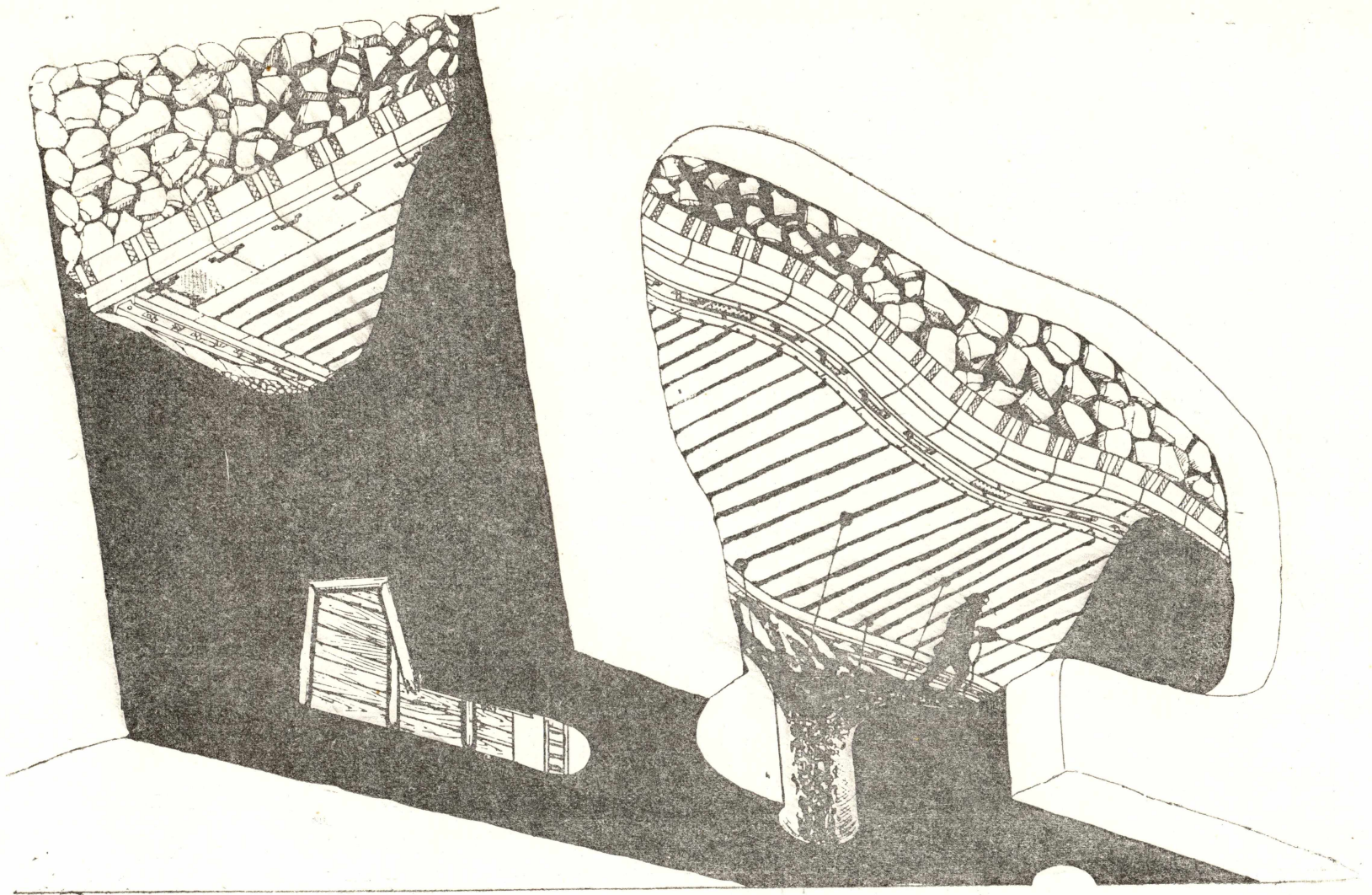
Рис. 1. Эластичный бессекционный щит
