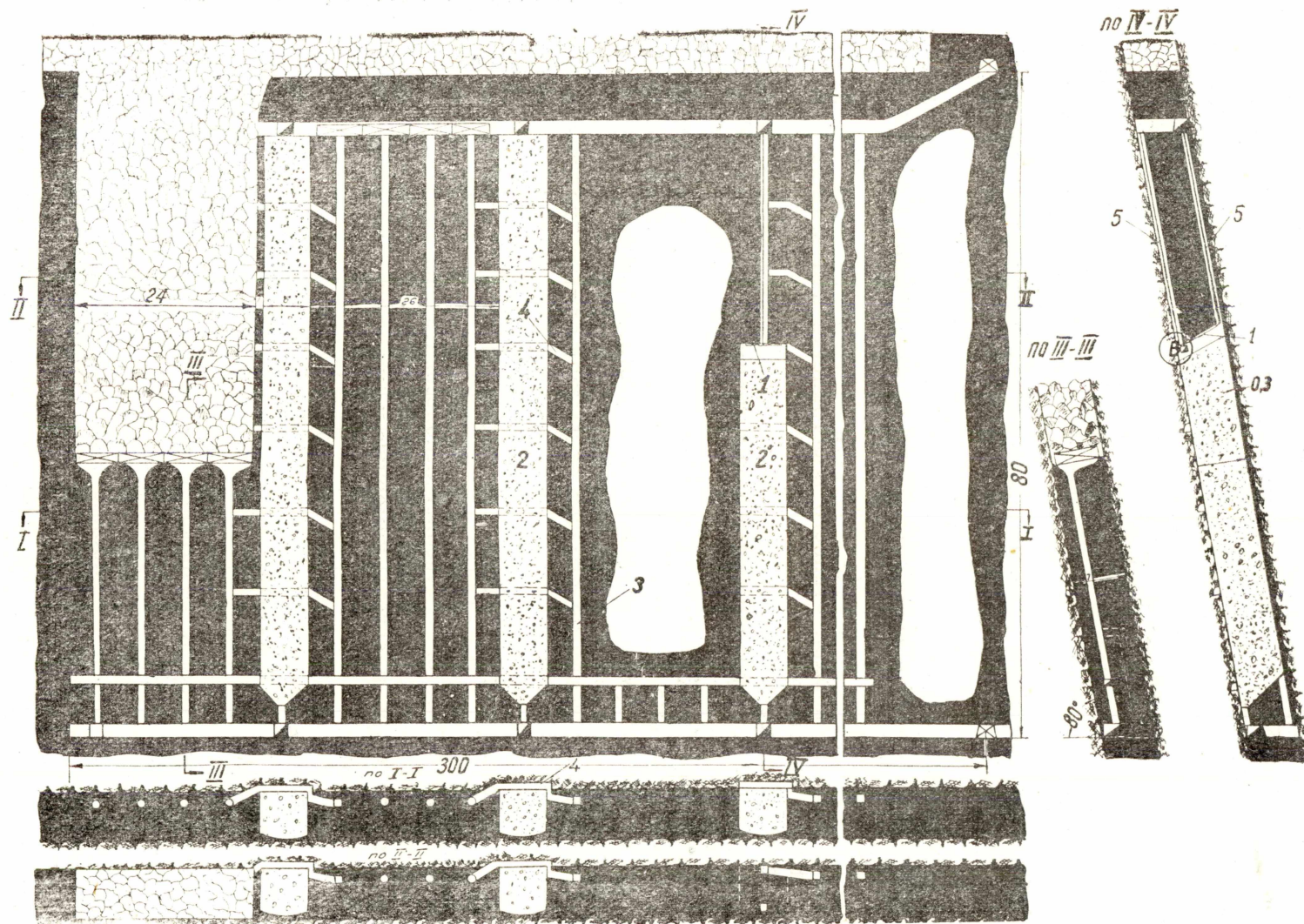
Рис. 12. Комбинированная система разработки мощных крутопадающих пластов (камерно-щитовая)
