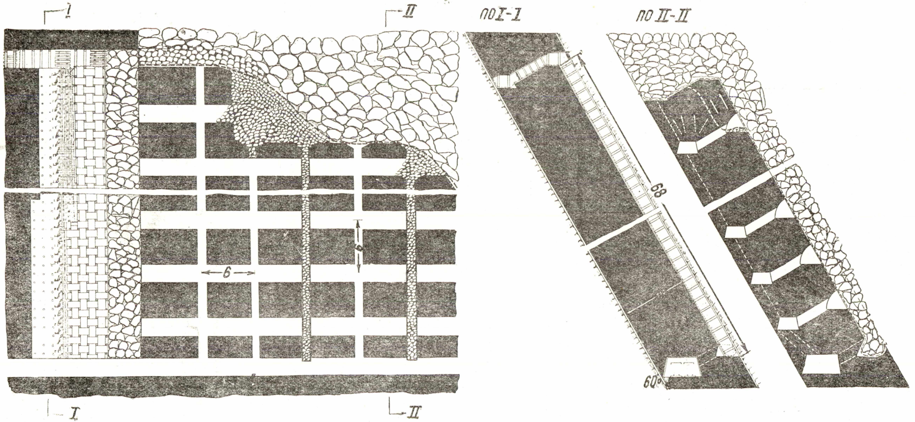
Рис. 11. Система разработки отступающим забоем под гибким перекрытием
