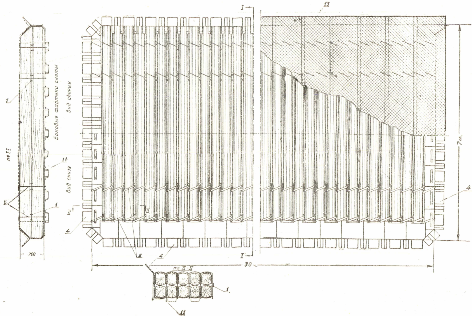
Рис. 2. Эластичный бессекционный щит из сдвоенных балок
