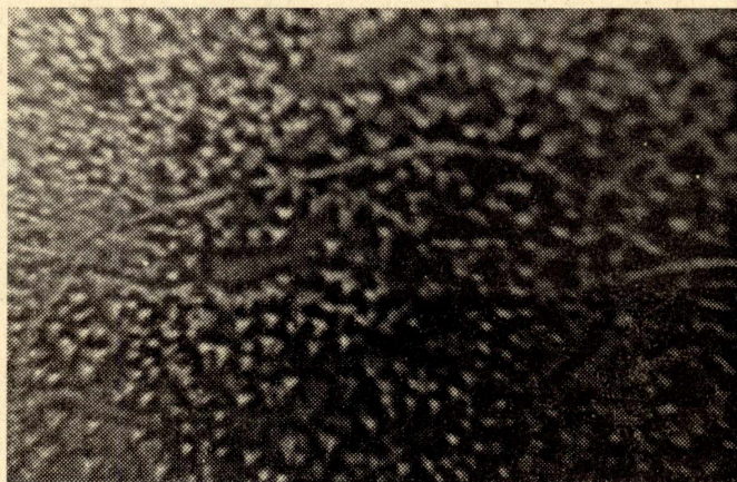
Рис. 2 б. Рельеф травленной по- верхности (III) природного бес- цветного флюорита, усеянный большим числом выступающих трехгранных вершин кубов раз- мером 0,005—0,001 мм
