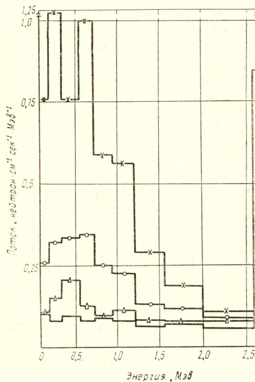
Рис. 2. Энергетическое распределение потока нейтронов, прошедших через двухслойный барьер полиэтилен — железо. Толщина полиэтилена 10 см. Толщина железа «— \Delta —» 1 см, «— \triangle —» 2 см, «— \circ —» 5 см, «— \times —» 10 см.
