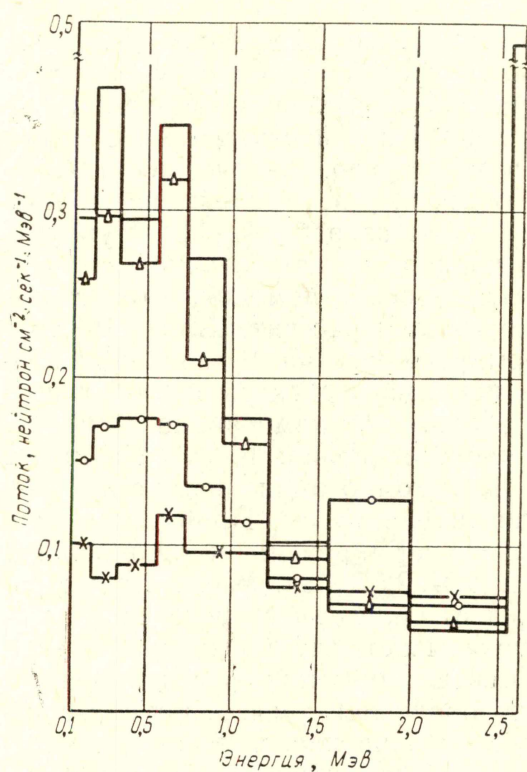
Рис. 1. Энергетическое распределение потока нейтронов, прошедших через двухслойный барьер железо — полиэтилен. Толщина железа 10 см. Толщина полиэтилена «— \Delta —» 1 см, «— \triangle —» 2 см, «— \circ —» 5 см, «— \times —» 10 см.
