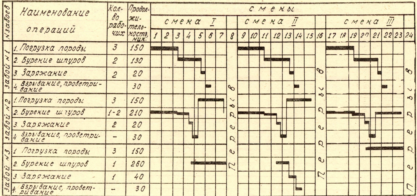
Рис. 3. Циклограмма работ при проведении выработок тремя забоями
