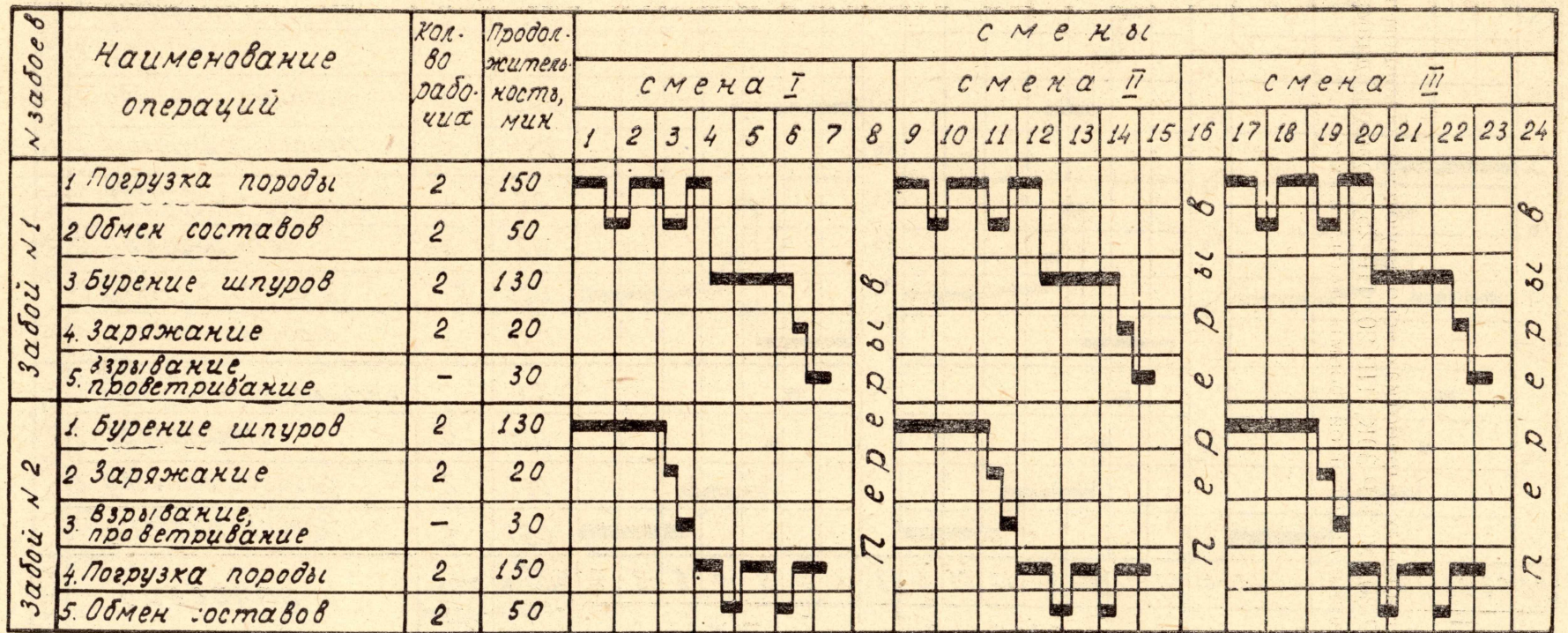
Рис. 2. Циклограмма работ при проведении выработок двумя забоями
